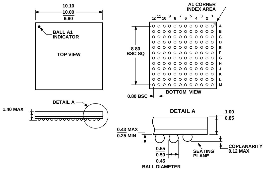
图72. 144引脚CSP_BGA芯片级封装 (BC-144-1)
