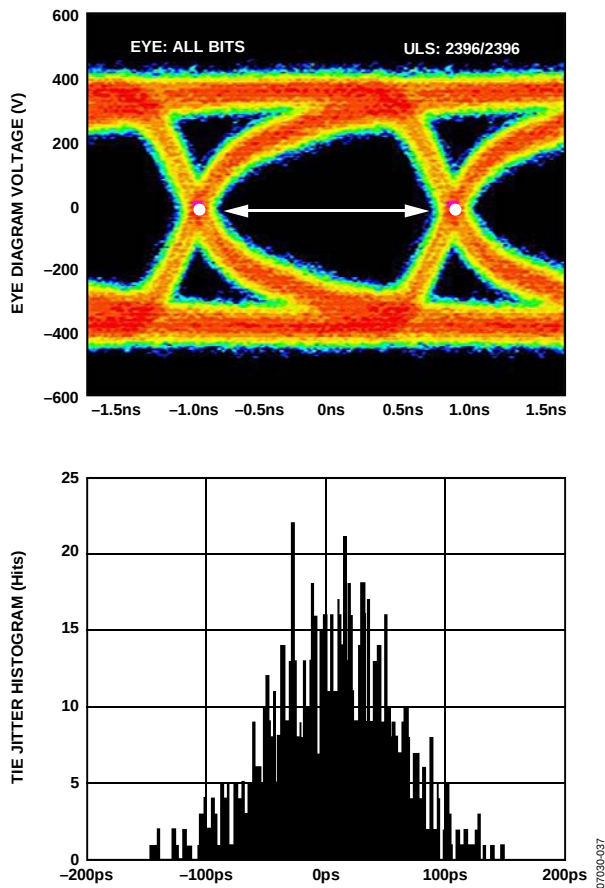
图67. LVDS输出的数据眼(ANSI-644模式， 100 Ω端接电阻，走线长度大于24英寸，标准FR-4)
