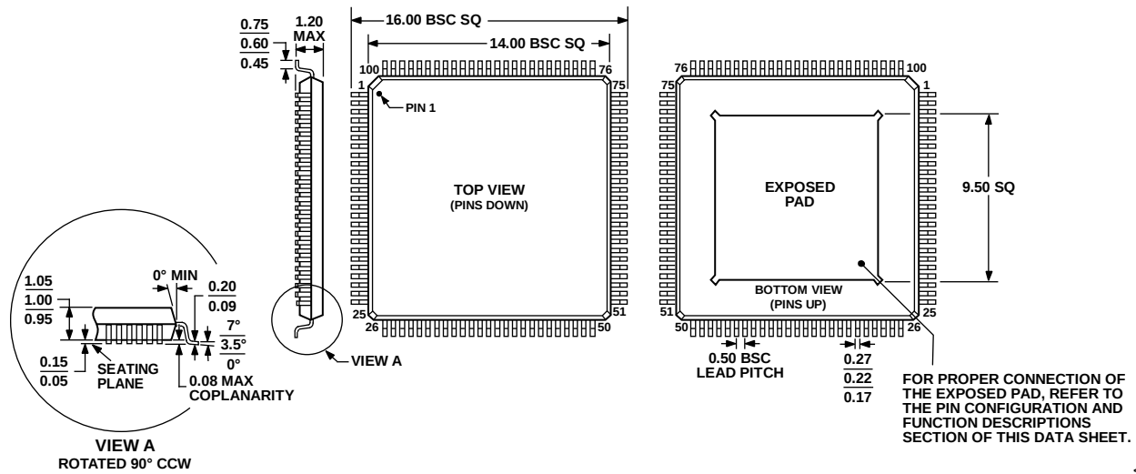
图71. 100引脚裸露焊盘超薄四方扁平封装 [TQFP_EP] (SV-100-3)
