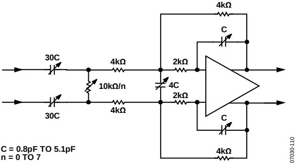
图54. 滤波器原理示意图
