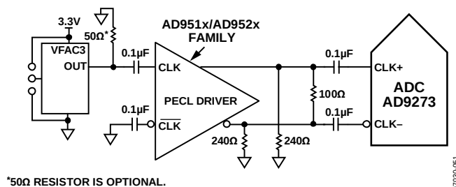
图56. 差分PECL采样时钟
