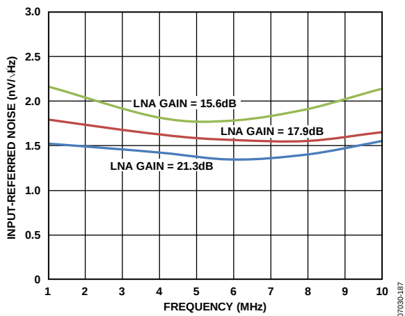
图14. 短路, 折合到输入的噪声与频率的关系, PGA 增益 = 30 dB, GAIN+ = 1.6\text{ V}
