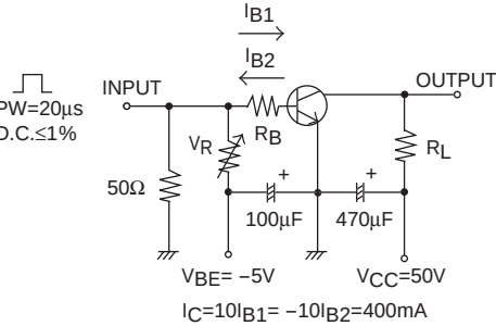
2SC4488
