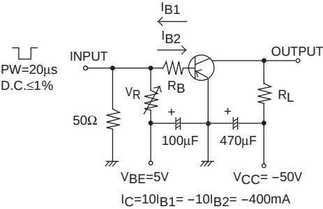
2SA1708
