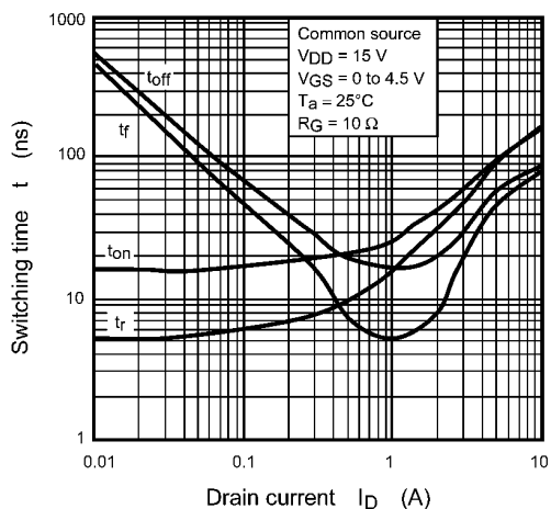
Fig. 7.11 t - I_D
