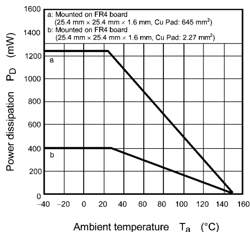
Fig. 7.14 P_D - T_a
