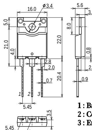
外形図 2174A (unit : mm)
