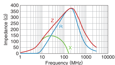
MPZ2012S331ATD25
