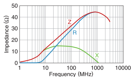
MPZ2012S331ATD25
