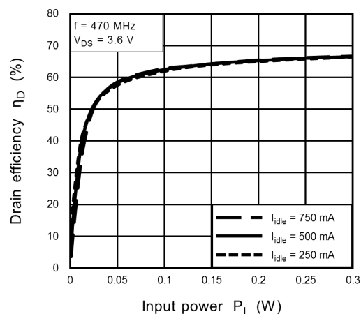
Fig. 8.4 \eta_D - P_I
