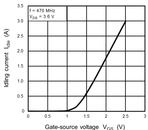
Fig. 8.5 I_{idle} - V_{GS}
