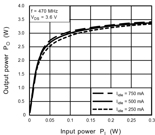
Fig. 8.3 P_O - P_I
