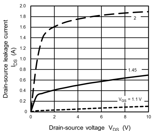
Fig. 8.6 I_{DS} - V_{DS}
