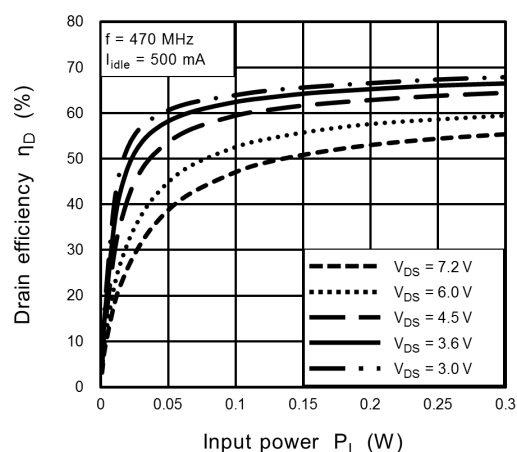
Fig. 8.2 \eta_D - P_I
