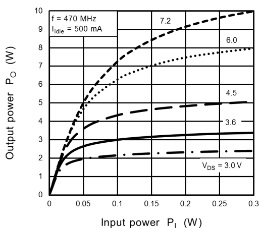
Fig. 8.1 P_O - P_I
