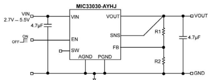
Figure 1. MIC33030-AYHJ Schematic
