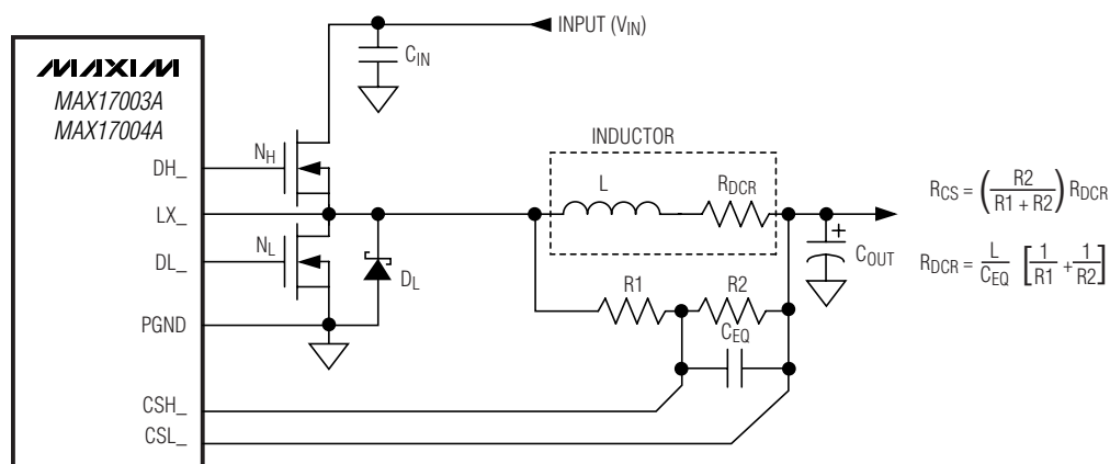
B) LOSSLESS INDUCTOR SENSING
