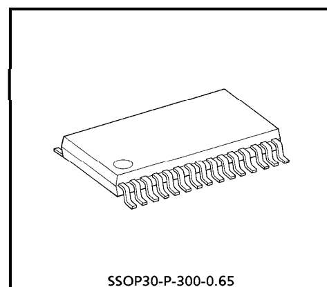
SSOP30-P-300-0.65
