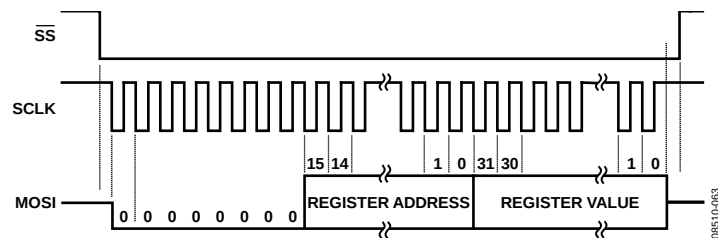
图90. 32位寄存器的SPI写操作
