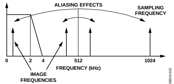
图32. 混叠效应
