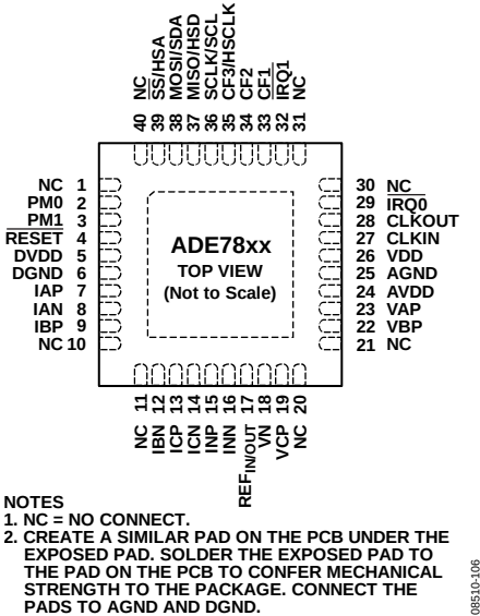
图9. 引脚配置
