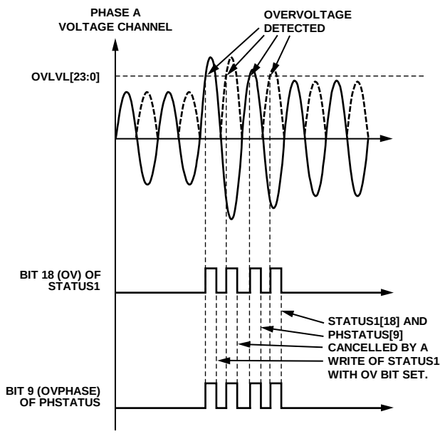
图52. 过压检测
