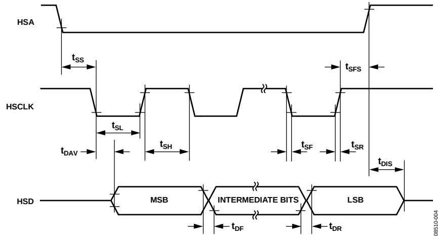
图7. HSDC接口时序
