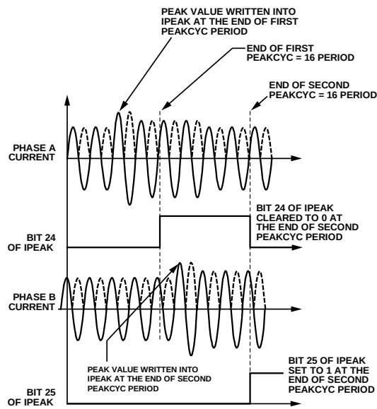
图51. 峰值电平检测
