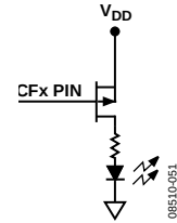
图76. CFx引脚推荐连接方式
