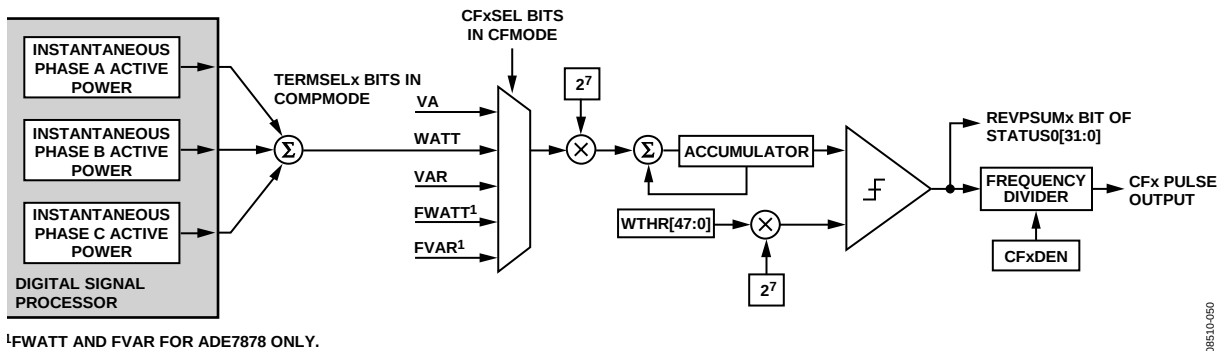
图75. 电能频率转换
