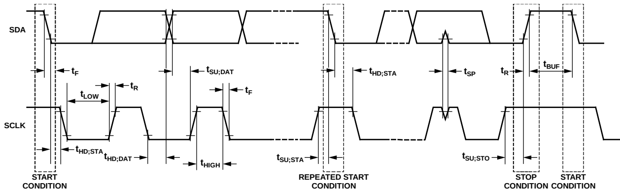
图5. I²C兼容接口时序
