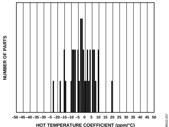
图58. 基准电压源漂移直方图(25°C至85°C)
