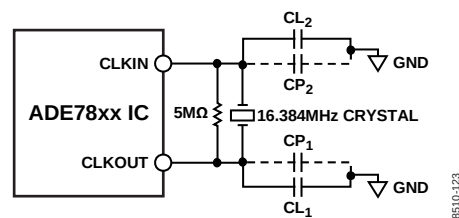
图98. 晶振电路
