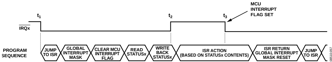
图84. 中断管理
