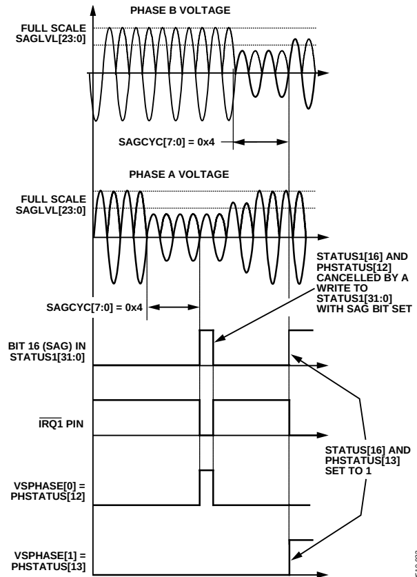
图49. SAG检测
