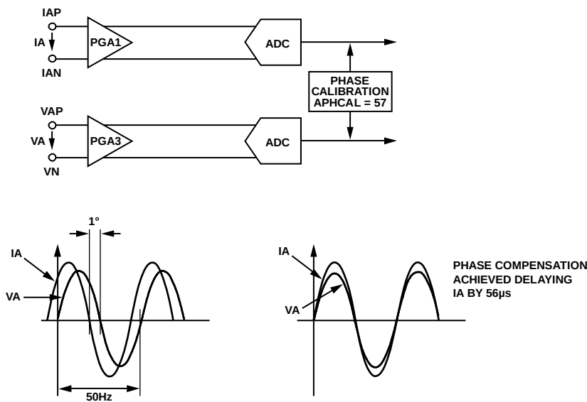
图55. 电压通道上的相位校准
