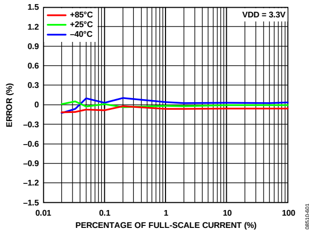
图10. 内部基准电压源和积分器关闭(增益 = +1, 功率因数 = 1)时整个温度范围内的总有功功率误差(以读数百分比形式表示)
