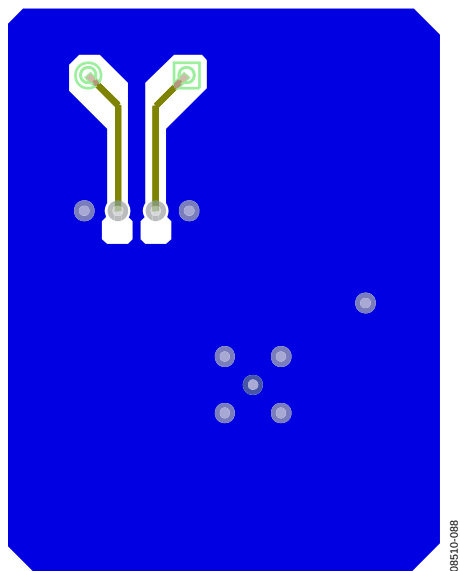
图97. ADE7878底层印刷电路板
