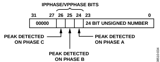
图50. IPEAK[31:0]和VPEAK[31:0]寄存器的组成成分
