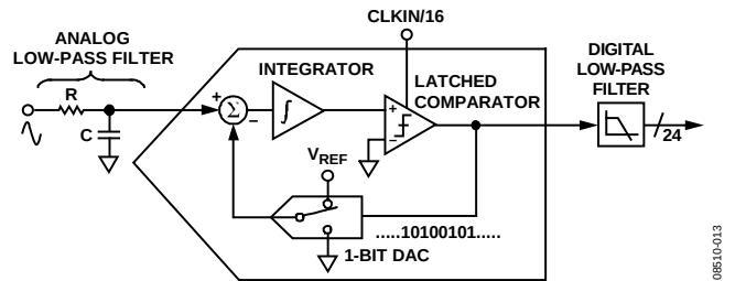
图30. 一阶 \Sigma - \Delta 型ADC
