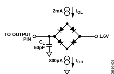
图 8. 时序规格的负载电路
