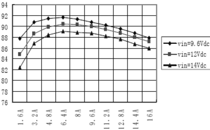
Vout 5V
