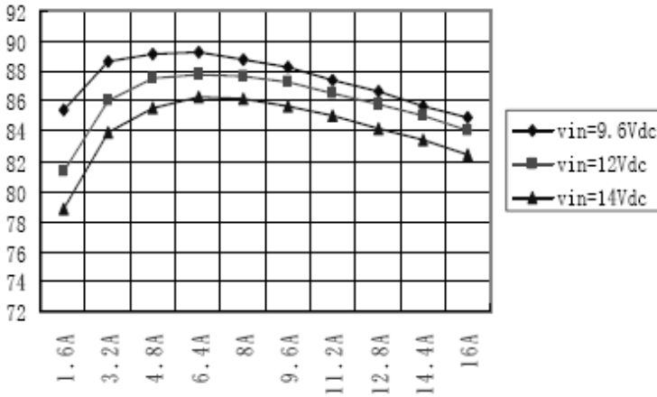
Vout 2.5V
