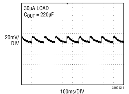
V_{OUT} Ripple
