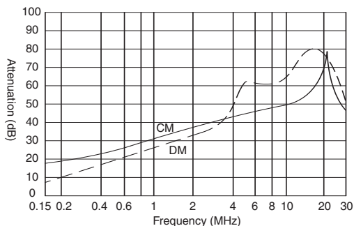
PLF-6DZ2R
