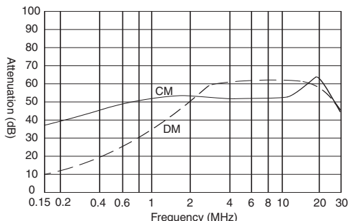
PLF-6DZ2R
