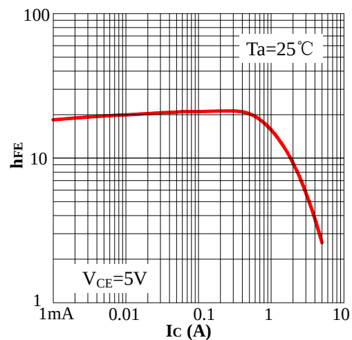
Fig2 h_{FE} - I_C
