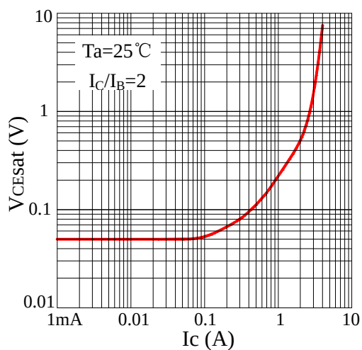
Fig3 V_{CEsat} - I_C
