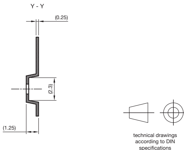
Fig. 13 - Taping
