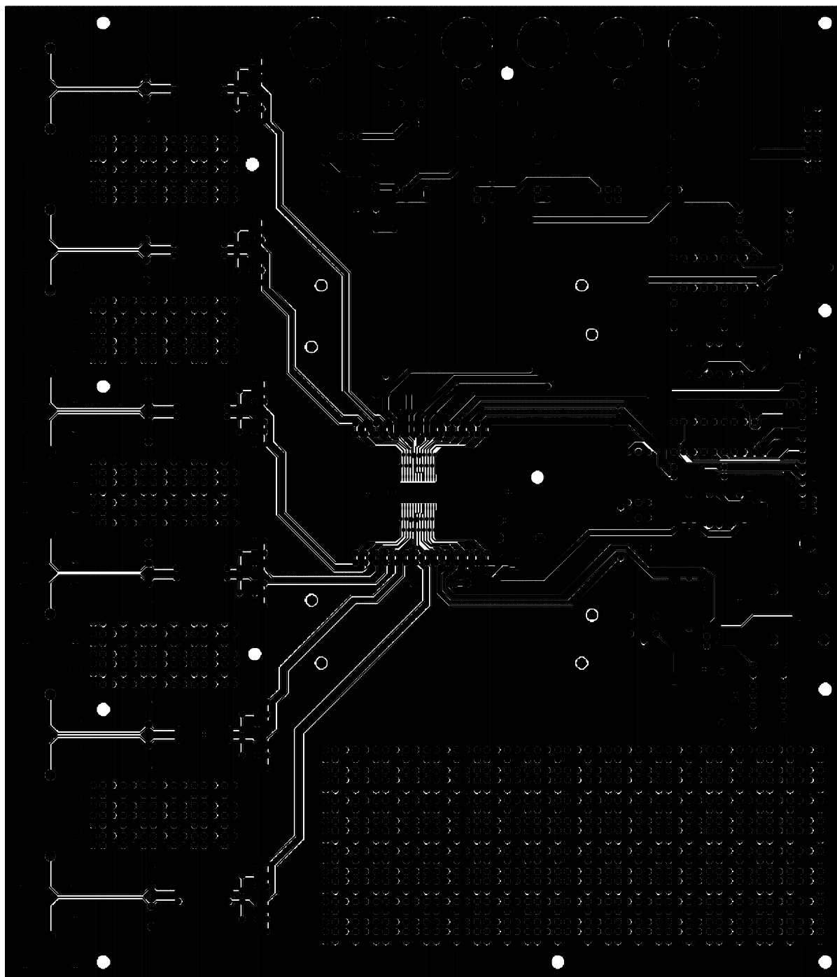
TOP SIDE
