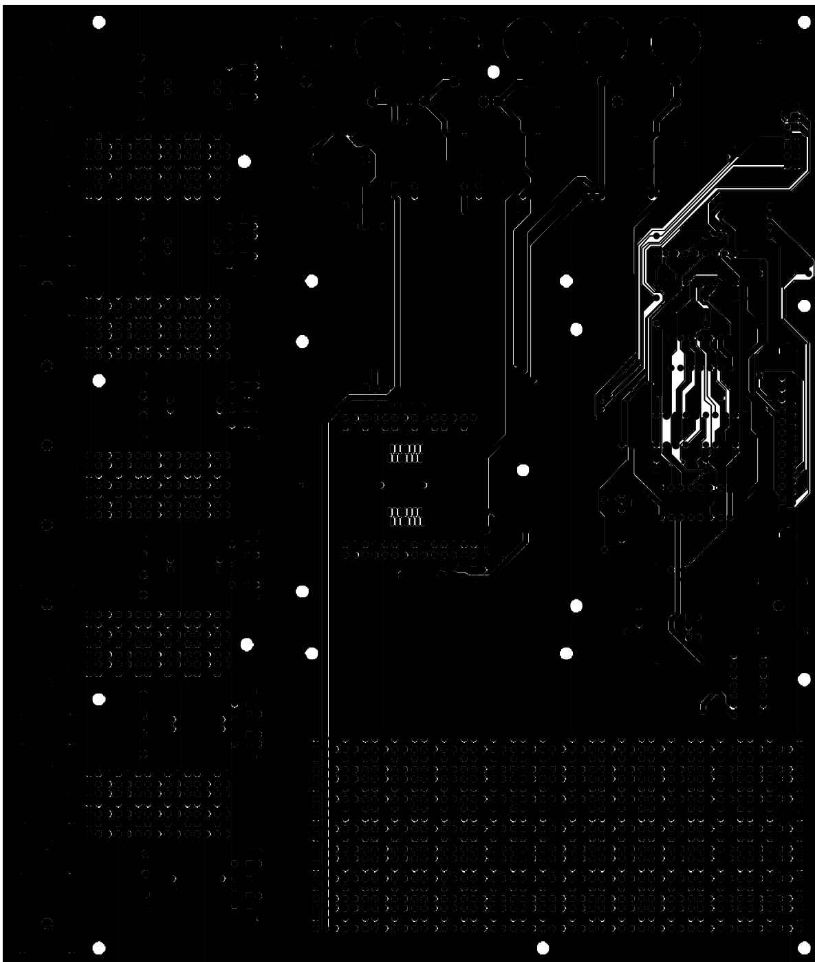
BOTTOM SIDE
