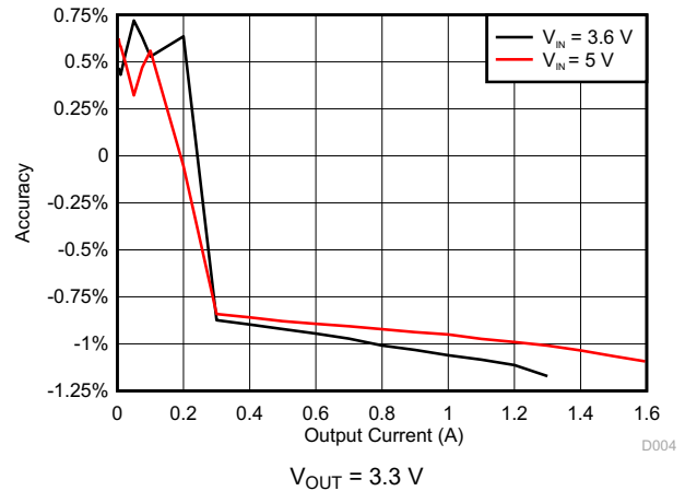
图 7-4. DCDC4 Accuracy
