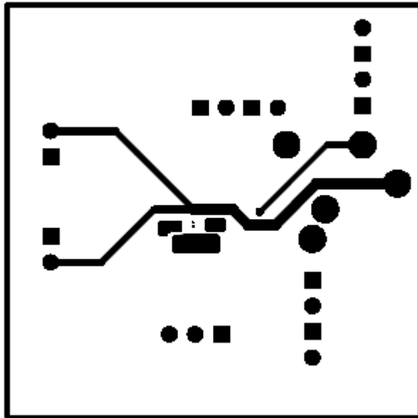
Figure 24. Bottom Layer
