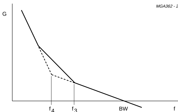
Fig.21 Motor servo mode diagram.
