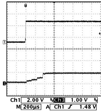
V_{OUT} = 1.2\text{ V} 1-A Load
