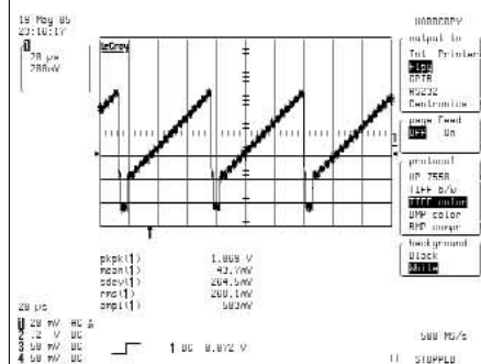
Ref.6 Y signal input : IC200, #62
