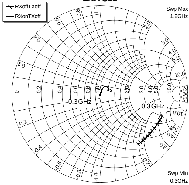
LNA S11
