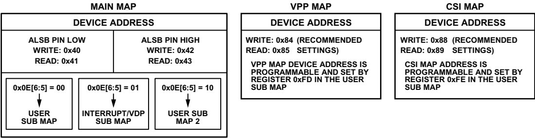
图14. 寄存器映射和子映射访问
