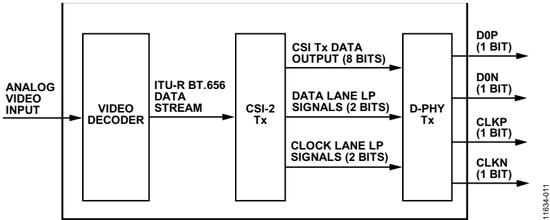
图10. ADV7280-M的MIPI CSI-2输出级
