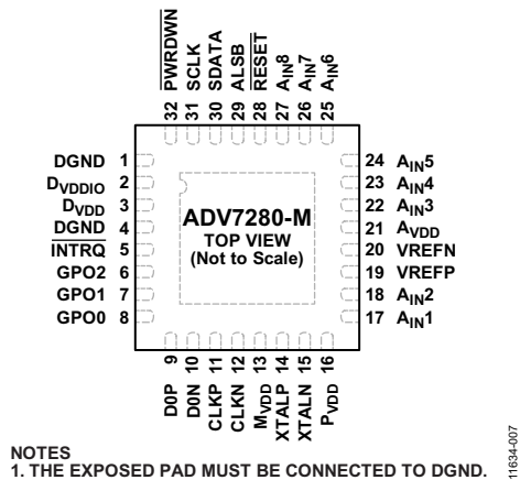
图7. ADV7280-M引脚配置
