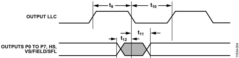
图4. ADV7280像素端口和控制输出时序图
