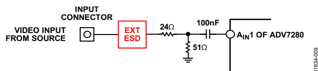
图9. 输入网络
