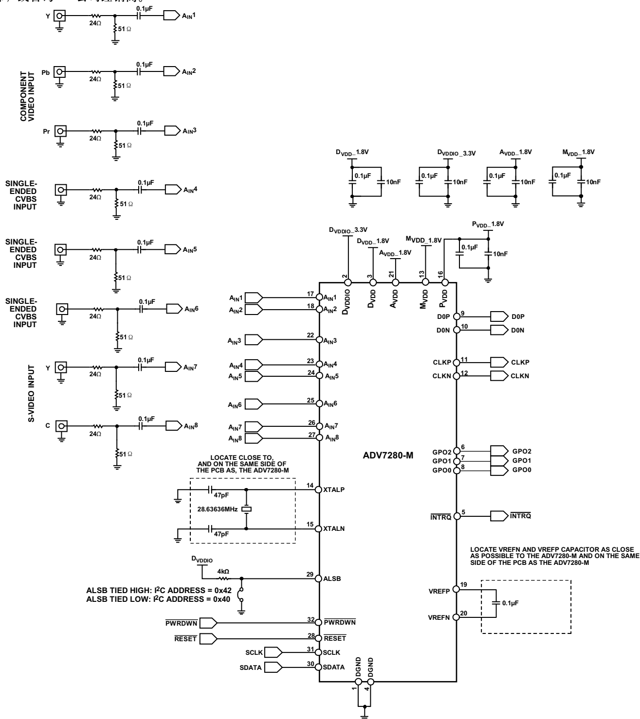
图17. ADV7280-M典型连接图
