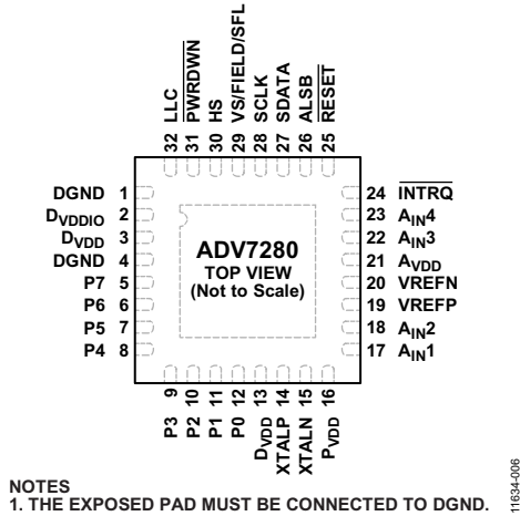
图6. ADV7280引脚配置
