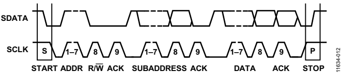
图12. 总线数据传输
