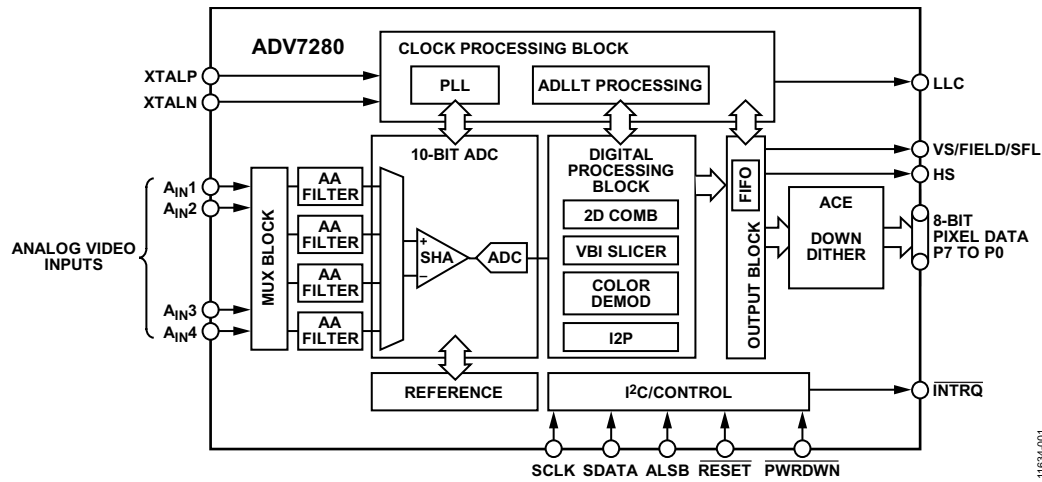
图1. ADV7280功能框图
