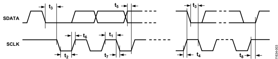
图5. I 2 C时序图
