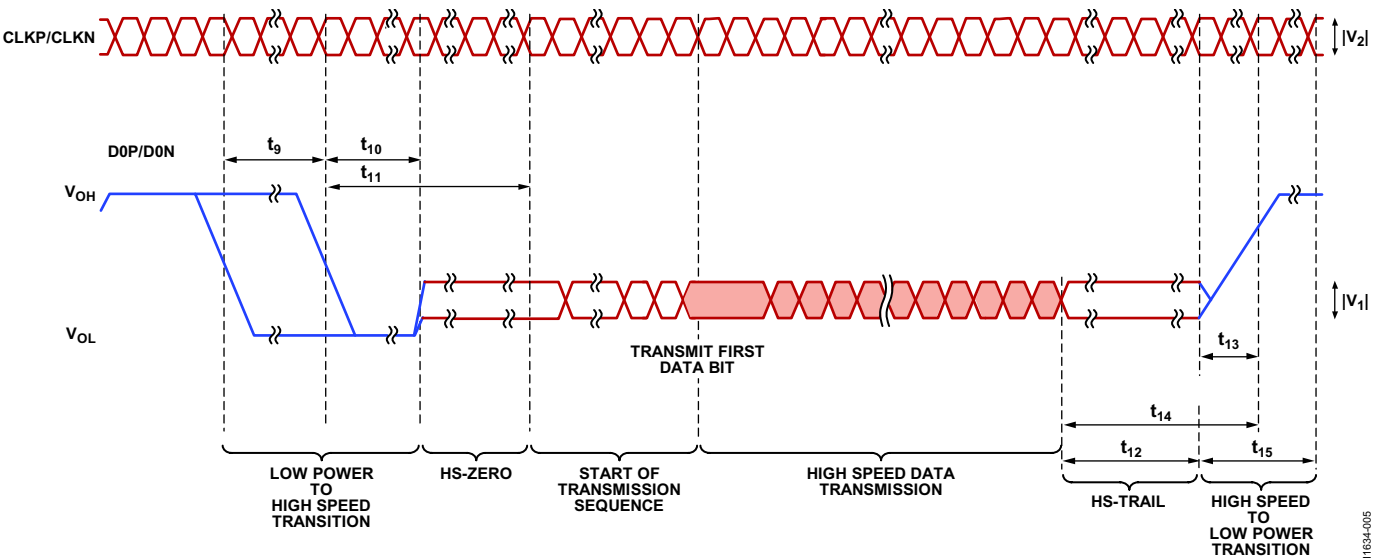
图3. ADV7280-M输出时序图(符合MIPI CSI-2规格)
