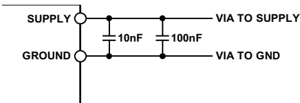
图15. 推荐的电源去耦
