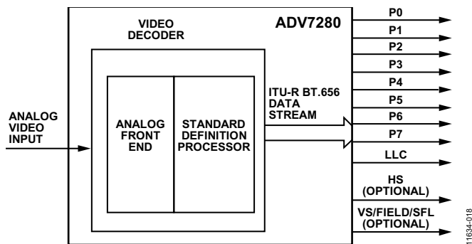
图11. ADV7280的ITU-R BT.656输出级
