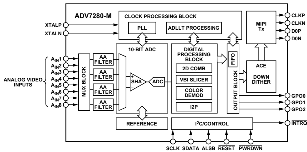
图2. ADV7280-M功能框图
