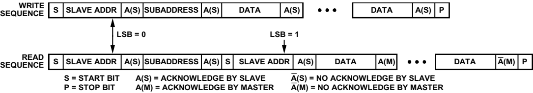
图13. 读取和写入序列
