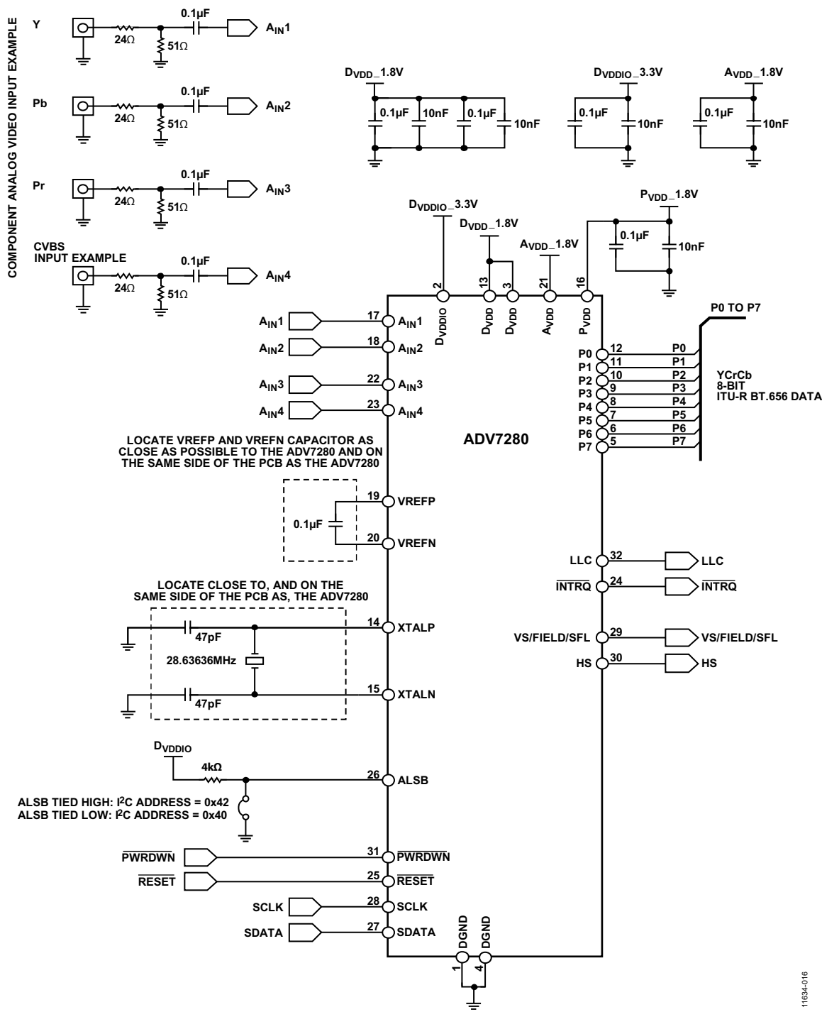
图16. ADV7280典型连接图
