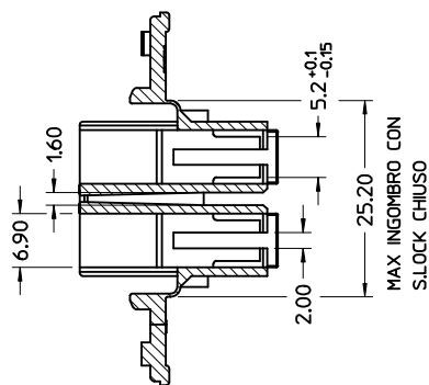
SEZ: C-C
