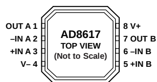
图2. 8引脚MSOP和8引脚SOIC_N封装
