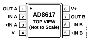
图2. 8引脚MSOP和8引脚SOIC_N封装
