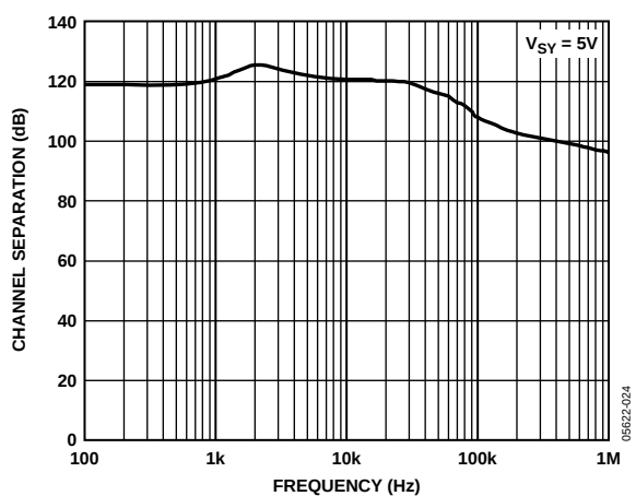
图26. 通道隔离度
