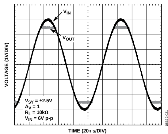
图23. 无相位反转
