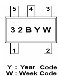
SOT-353 ( SC-70 )
