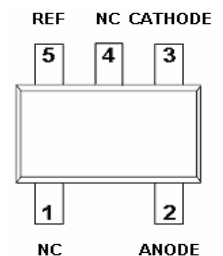
SOT-353 ( SC-70 )
