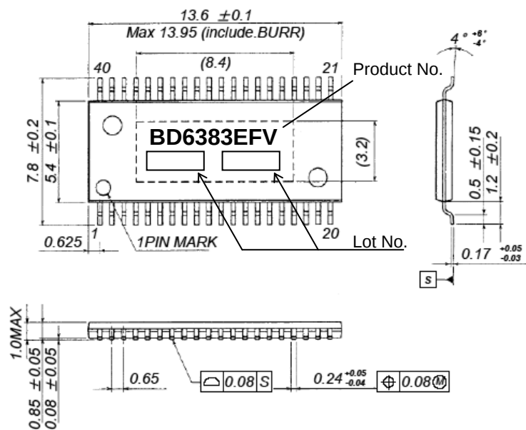
HTSSOP-B40 (Unit:mm)
