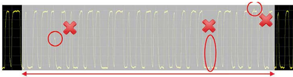
그림 9: 타사의 오실로스코프는 초당 50,000개의 파형을 지원합니다. 데드 타임이 길기 때문에 간헐적 이벤트를 캡처할 수 있는 확률이 낮습니다.
