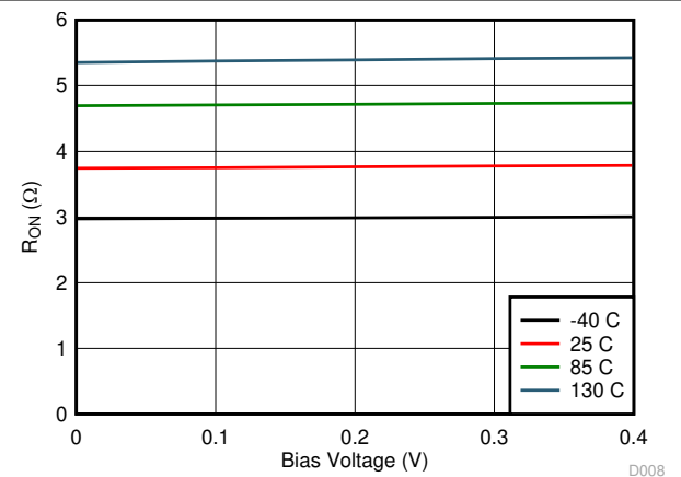
图 6-6. Data Switch R_{ON} vs Bias Voltage
