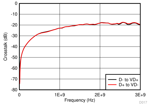
图 6-14. Data Switch Crosstalk
