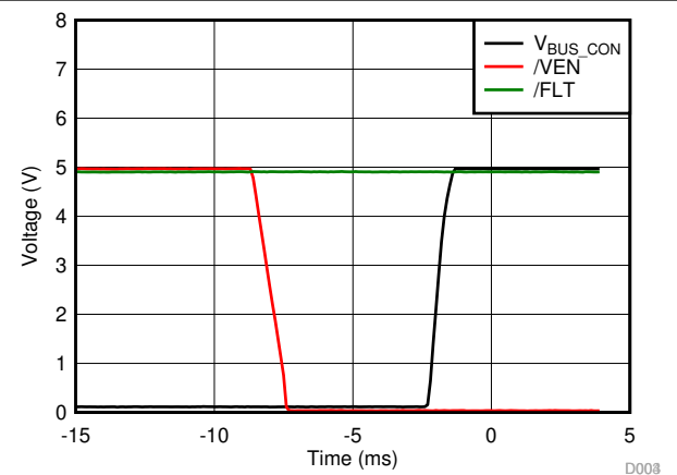
图 6-4. V_{BUS} t_{ON} Time
