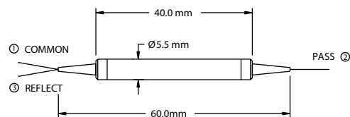
P2: 900 \mu m loose tube
