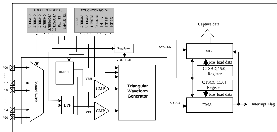
图 5-36 电容传感器框图
