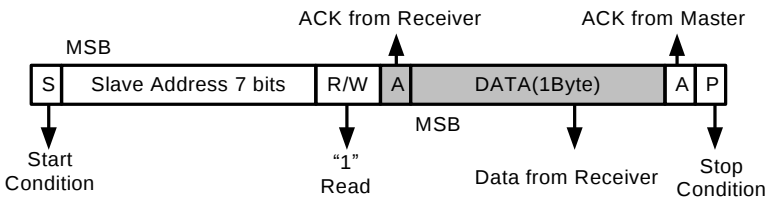
图 5-32 7-bits 地址读模式
