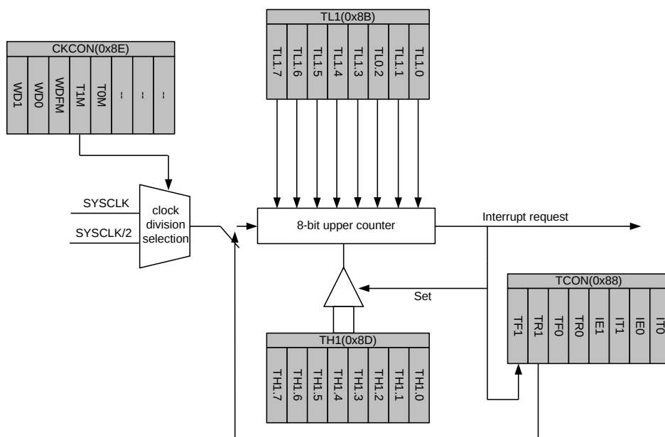
图 5-16 Timer 1 模式 2 示意图
