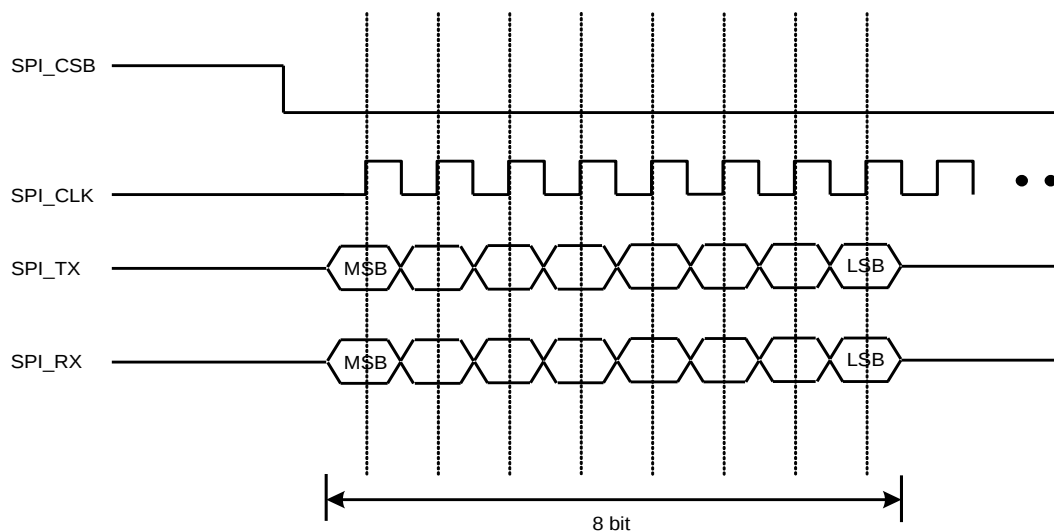
图 5-26 主模式, POLARITY=0, PHASE=0
