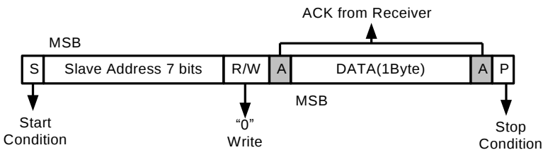
图 5-31 7-bits 地址写模式
