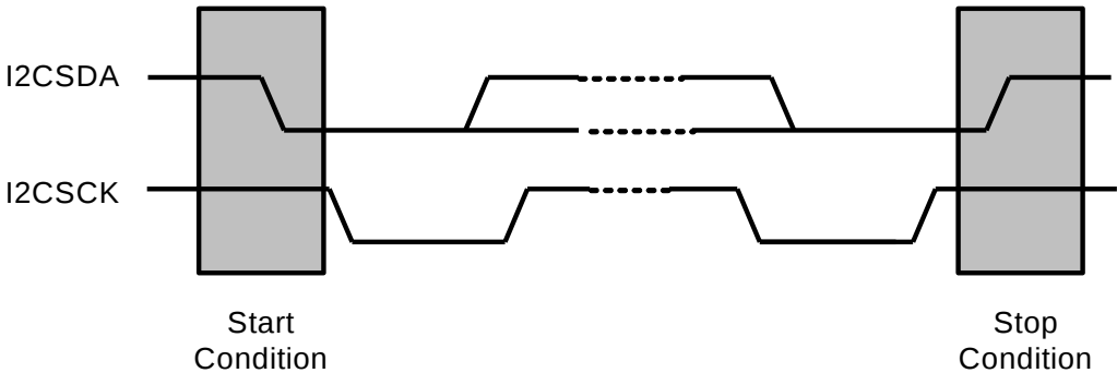
图 5-30 起始和停止条件
