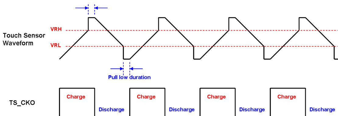
图 5-34 电容传感器输出频率时序图(EN_TRI = "0")
