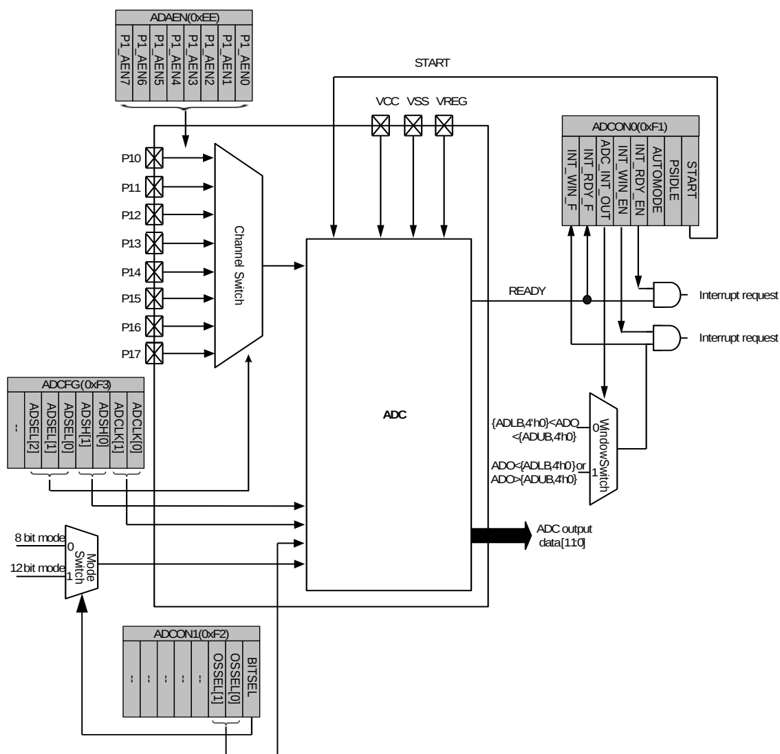
图 5-39 ADC 方框图
