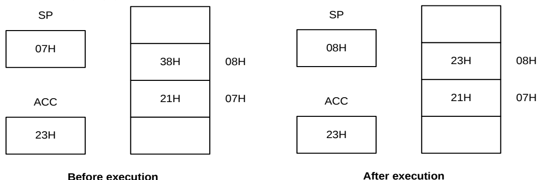
图 5-2 “PUSH A”指令的堆栈顺序
