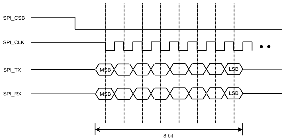
图 5-28 主模式, POLARITY=1, PHASE=0
