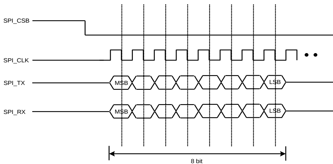
图 5-27 主模式, POLARITY=0, PHASE=1
