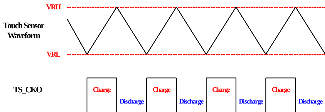
图 5-35 电容传感器三角波输出频率时序图(EN_TRI = "1")
