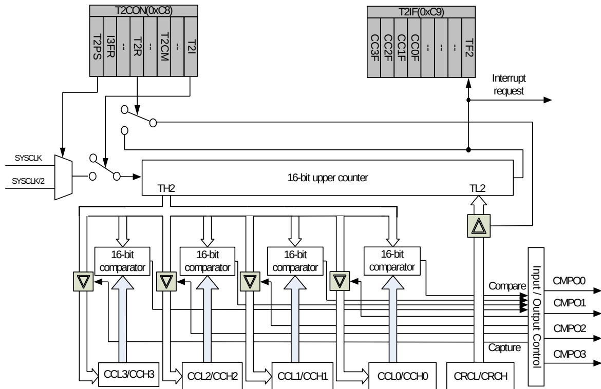
图 5-17 Timer 2 比较捕捉功能示意图
