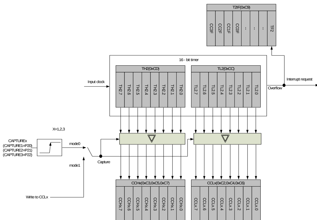
图 5-20 CCLx 和 CCHx (x=1,2,3) 的 Timer2 捕捉模式 0 示意图
