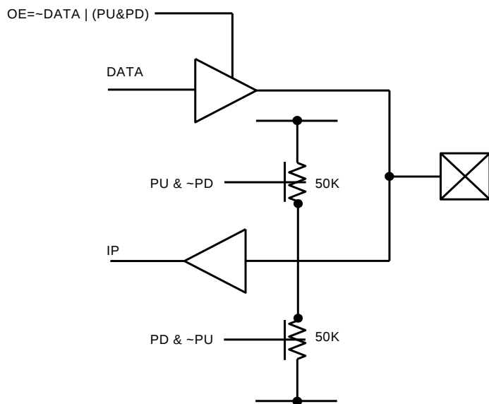
图 5-9 数字脚示意图
