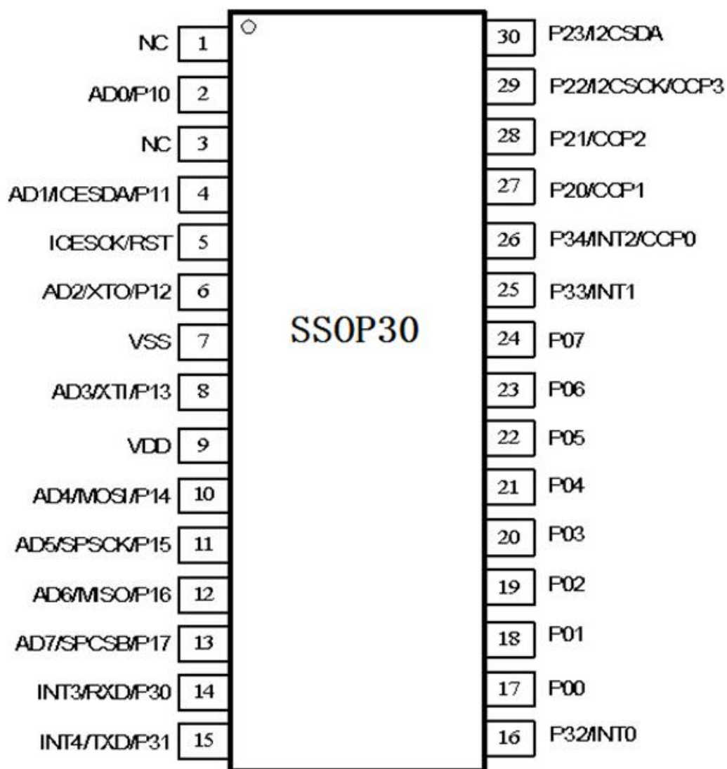
图 4-2 GPM8F3716B(SSOP30)脚位图
