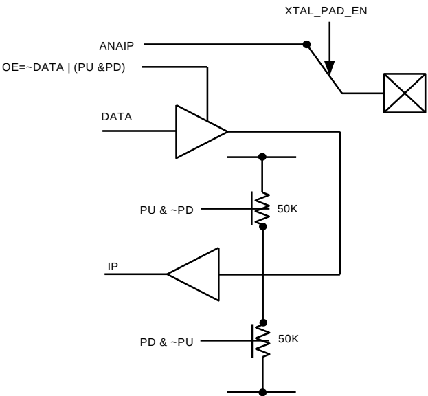
图 5-8 模拟脚示意图
