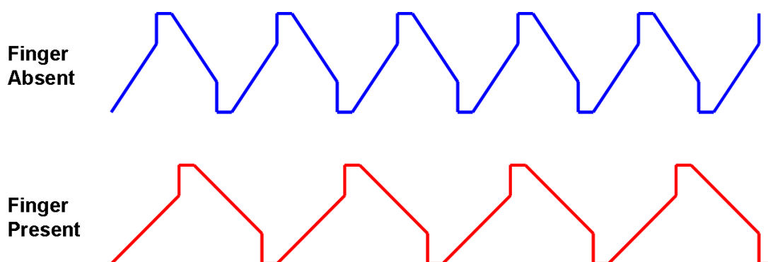
图 5-33 手指触碰和离开的时序状态图
