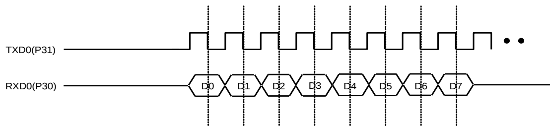
图 5-22 UART0 模式 0 发送时序图
