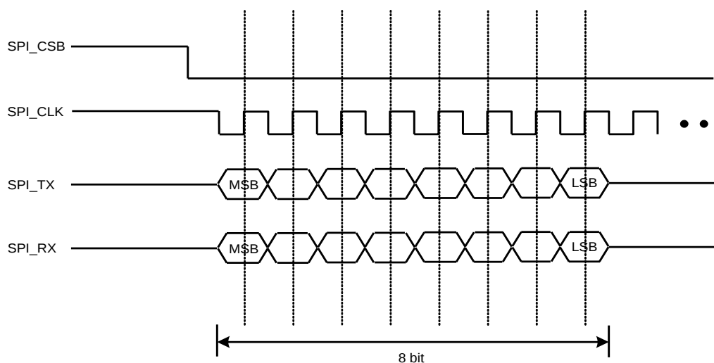
图 5-29 主模式, POLARITY=1, PHASE=1
