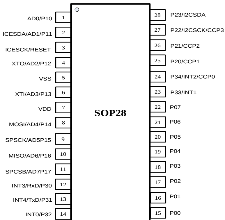
图 4-1 GPM8F3716B(SOP28)脚位图
