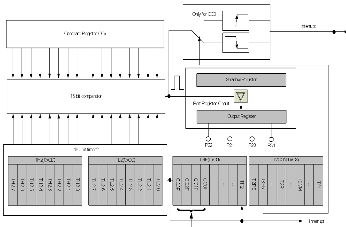
图 5-20 Timer 2 比较模式 1 示意图给出了 Timer 2 在比较模式 1 下的功能图。
