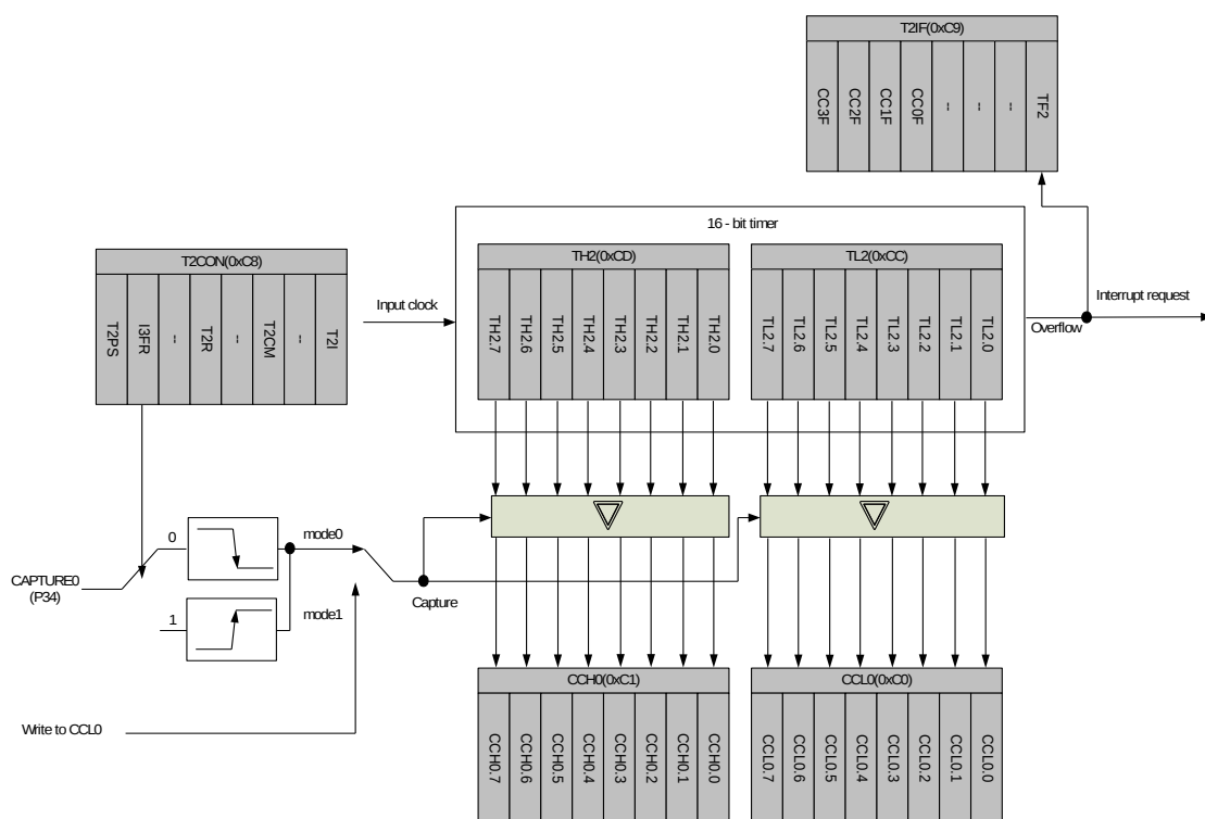
图 5-19 CCL0 和 CCH0 的 Timer2 捕捉模式 0 示意图
