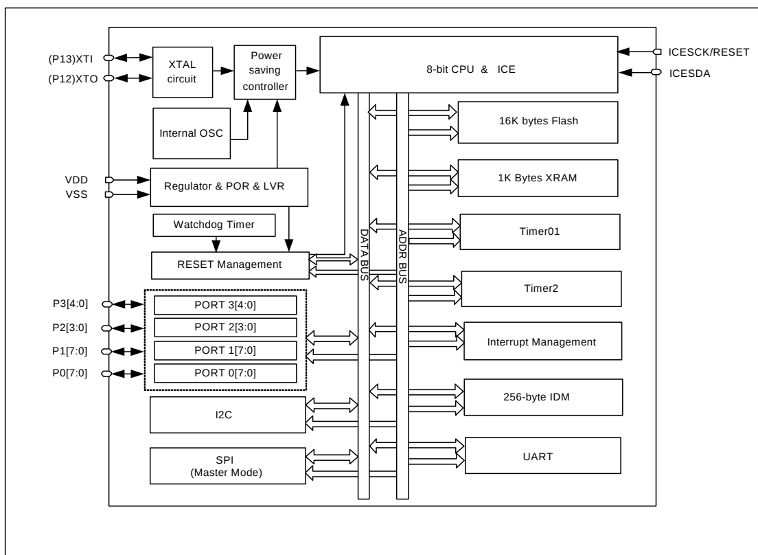
图 3-1 GPM8F3716B 框图
