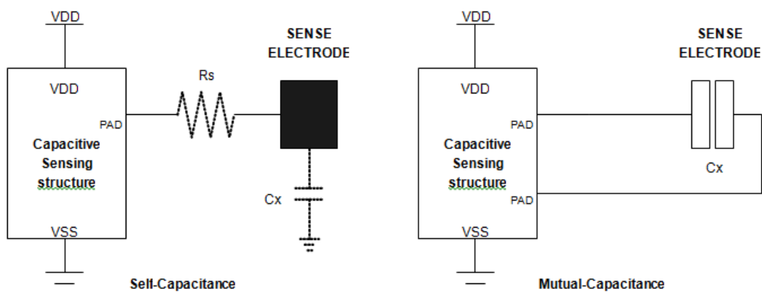
图 5-37 自感式电容感应和互感式电容感应
