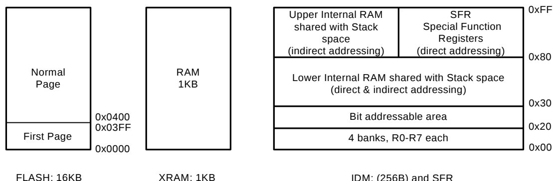
图 5-1 程序存储区和数据存储区
