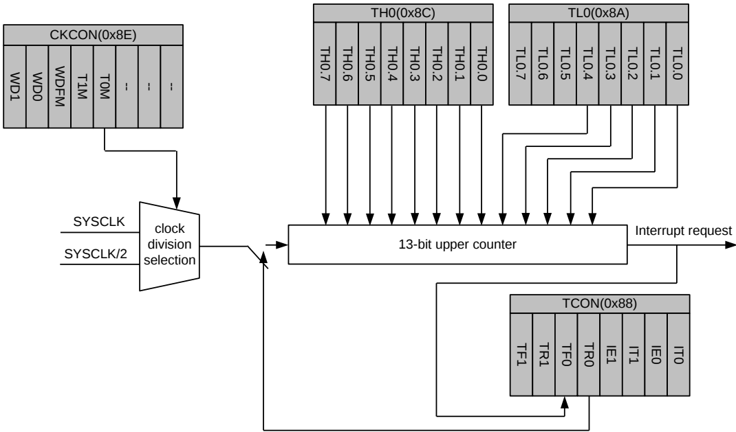
图 5-10 Timer 0 模式 0 示意图
