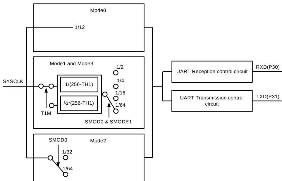
图 5-21 UART 模块示意图
