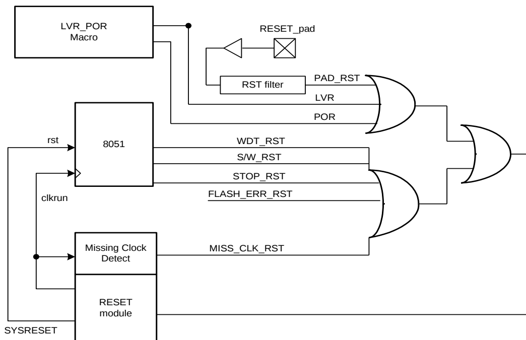
图 5-4 复位源
