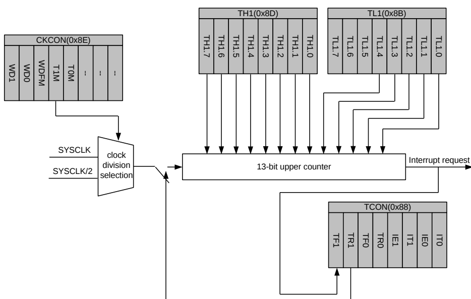
图 5-14 Timer 1 模式 0 示意图
