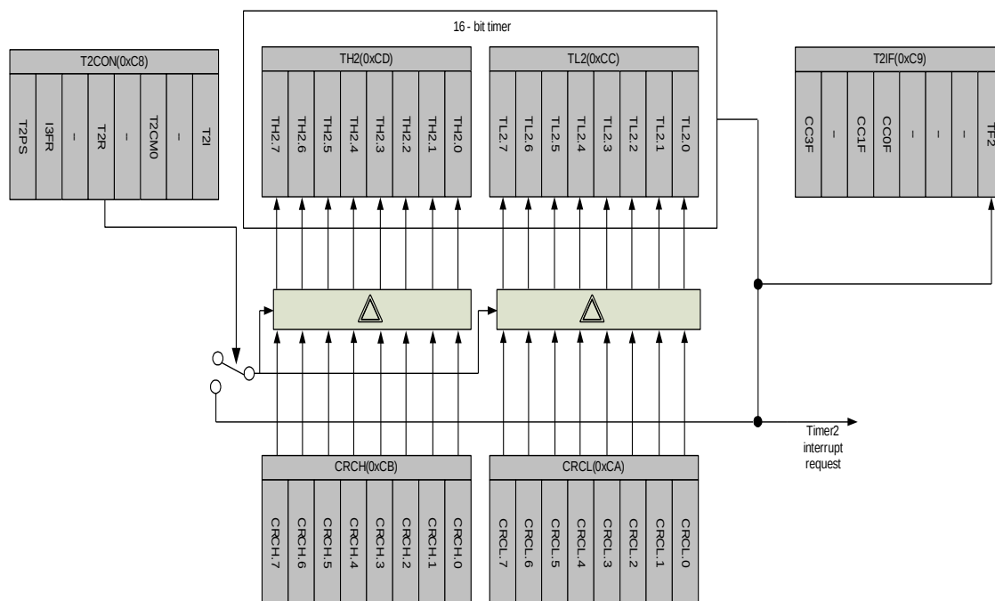
图 5-18 Timer 2 重载功能示意图
