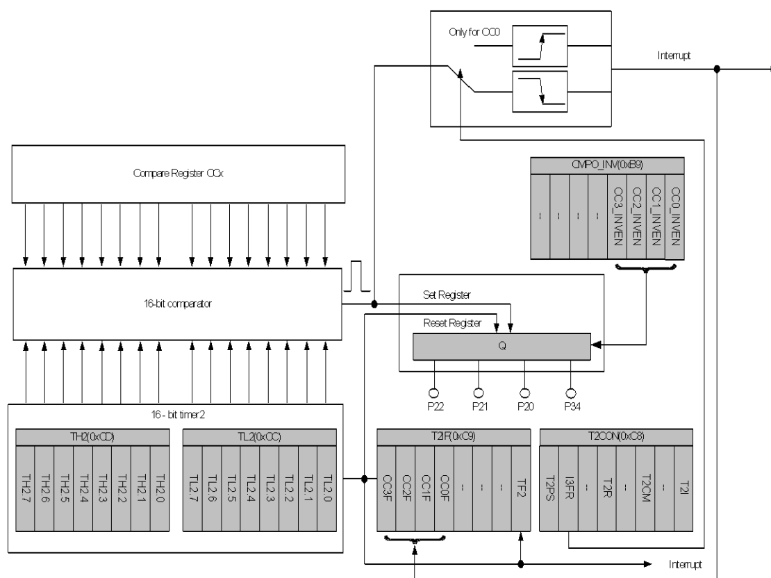
图 5-19 Timer 2 比较模式 0 示意图给出了比较模式的端口寄存器的功能示意图。P34/P20/P21/P22 端口寄存器由两个信号直接控制：定时器溢出和比较。
