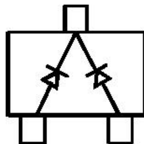
SOT-23 内部结构
