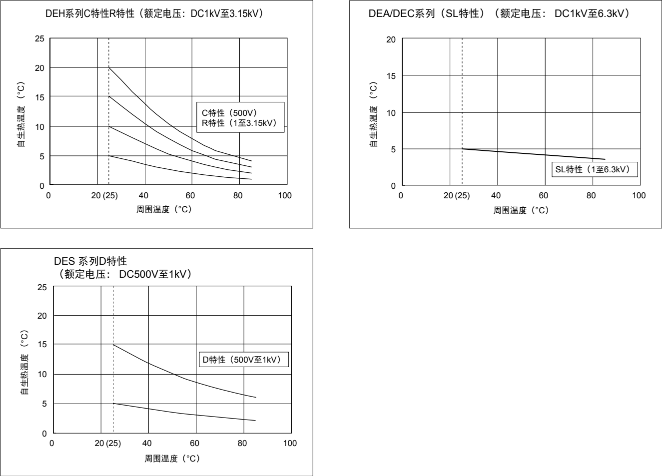
<图 2>自生热温度与周围温度的相关性
