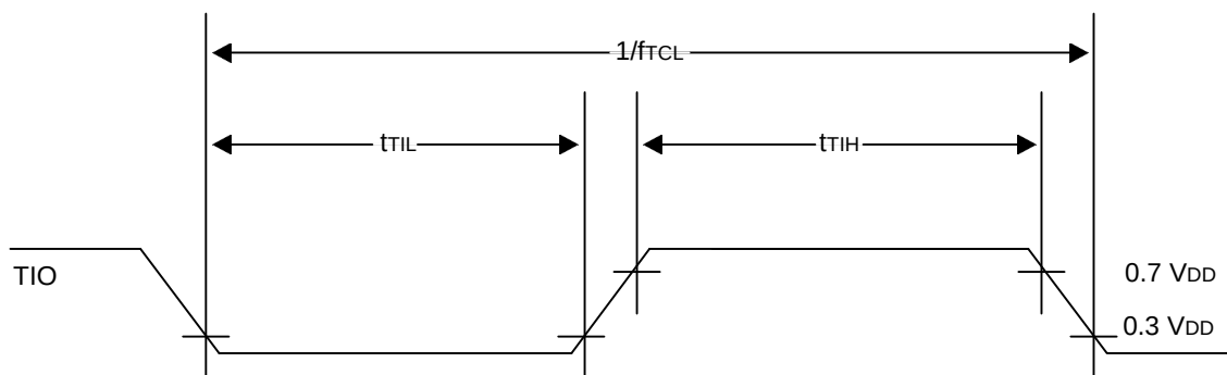
Figure 14-6. TIO Timing
