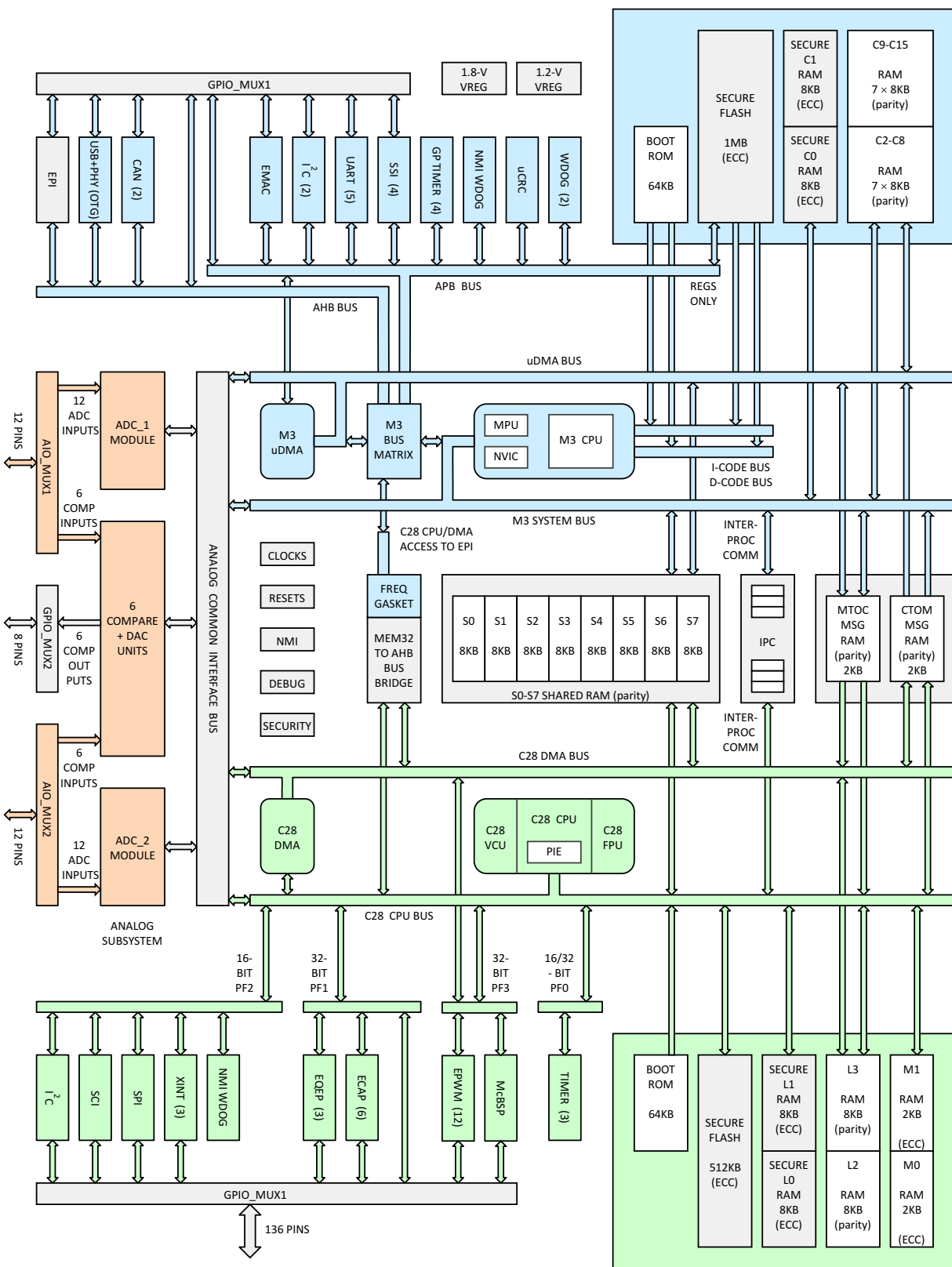
图 1-1. 功能框图
