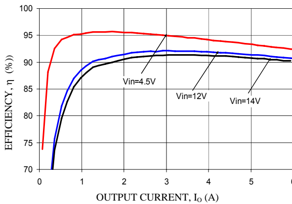
V_o=3.3V
