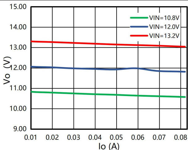
图5 输出电压 vs 输出电流 (VPS8701+VPT87DD-01B,12V to 12V/1W)
