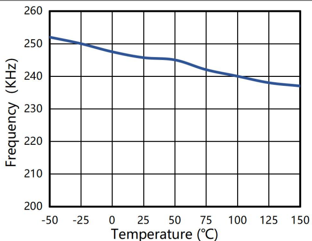
图 7 频率 vs 环境温度
