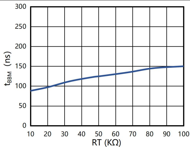
图 10 死区时间 vs RT
