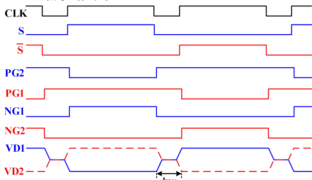
图 8.3.1 驱动时序图
