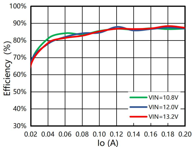
图2 转换效率 vs 输出电流 (VPS8701+VPT87DB-01B,12V to 5V/1W)
