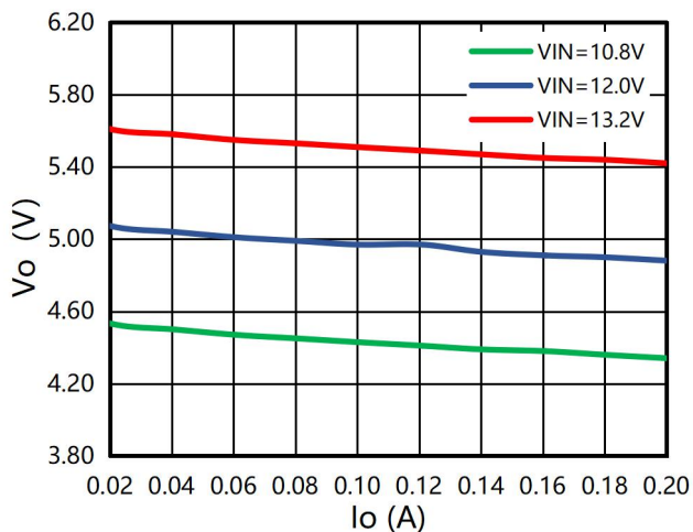
图1 输出电压 vs 输出电流 (VPS8701+VPT87DB-01B,12V to 5V/1W)
