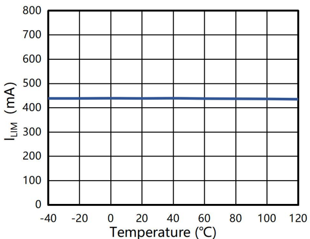
图 12 钳位电流 vs 环境温度
