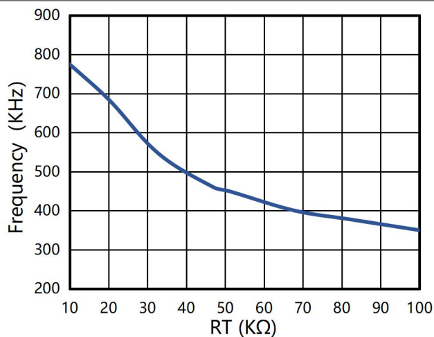
图 8 频率 vs RT
