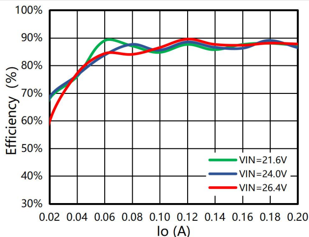
图4 转换效率 vs 输出电流 (VPS8701+VPT87FB-01B,24V to 5V/1W)
