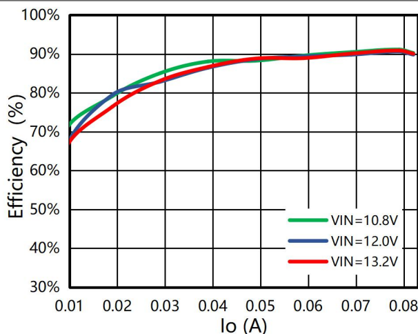
图6 转换效率 vs 输出电流 (VPS8701+VPT87DD-01B,12V to 12V/1W)
