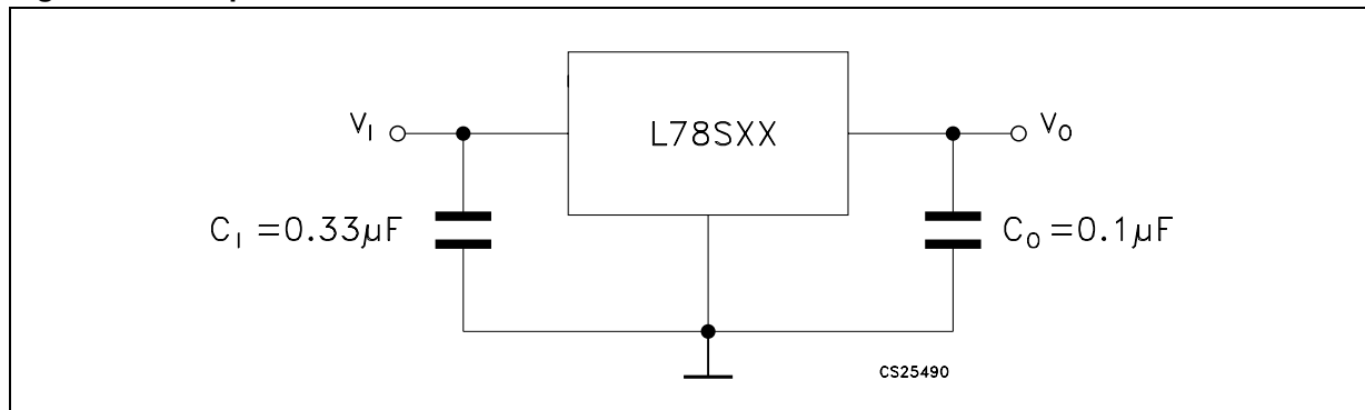
Figure 5. DC parameter
