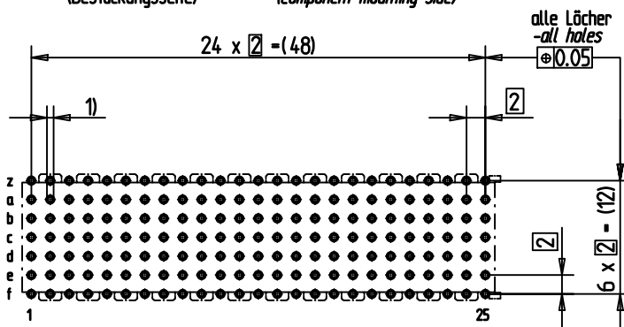
Lochbild für Leiterplatte (Bestückungsseite)
