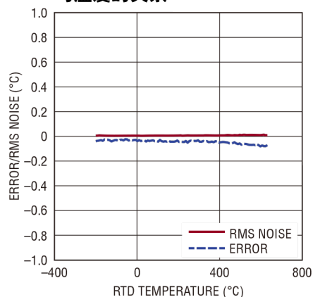
RTD PT-200 误差和 RMS 噪声与温度的关系
