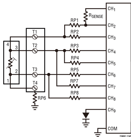
图 48. 带保护的多传感器四线式线 RTD 连接
