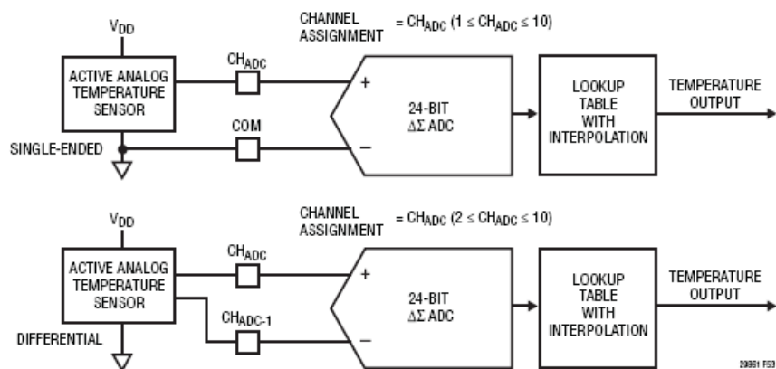
图 53. 有源模拟温度传感器通道分配约定
