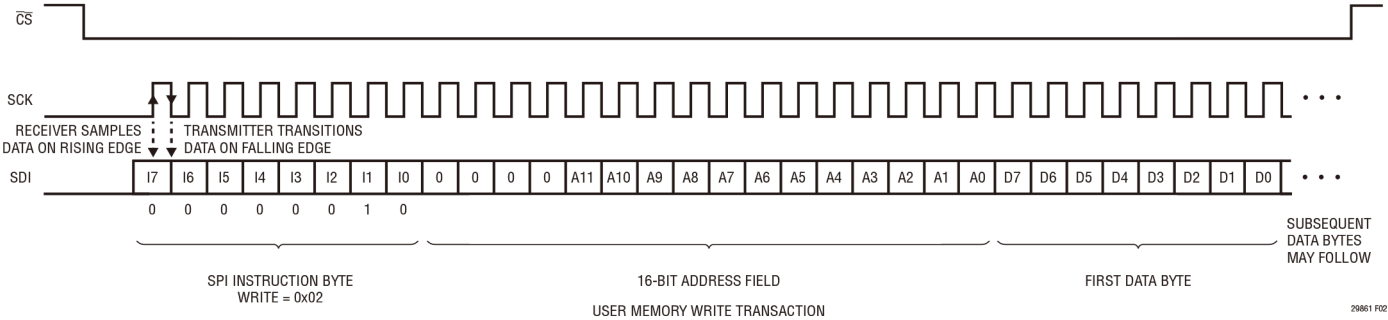
图 2. 存储器写操作
