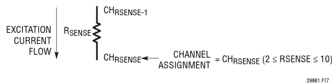
图 17. 四线式 RTD 检测电阻通道分配约定
