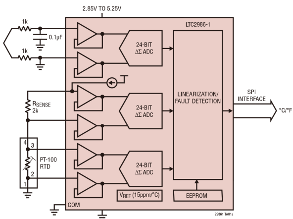
具有自动冷结点补偿功能的热点偶测量
