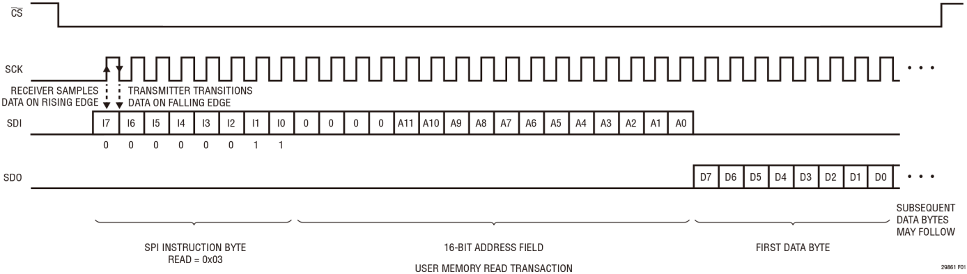
图 1. 存储器读操作
