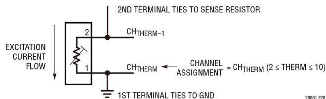
图 28. 差分热敏电阻通道分配约定
