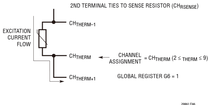
图 46. 热敏电阻开尔文电流模式通道分配约定 (G6 = 1)
