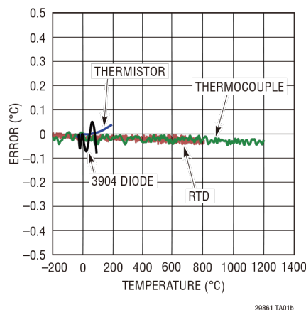
典型温度误差贡献
