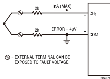
图 36. 带保护电阻的热电偶
