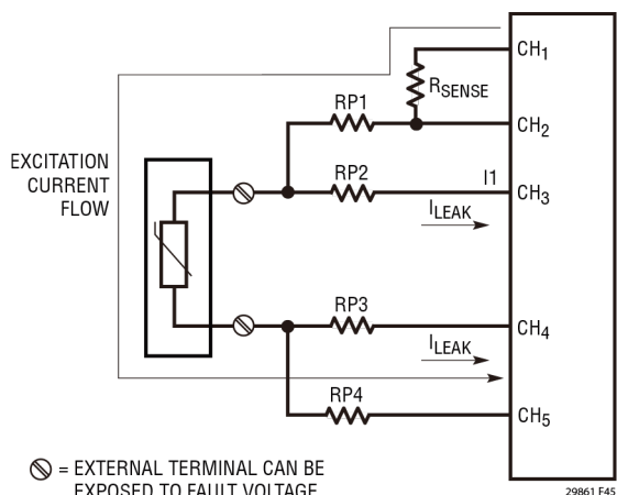
图 45. 热敏电阻开尔文电流源模式 (G6 = 1)
