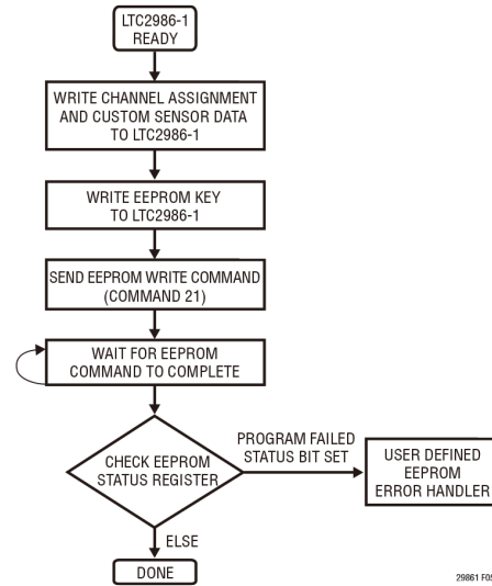
图 5. EEPROM 写操作
