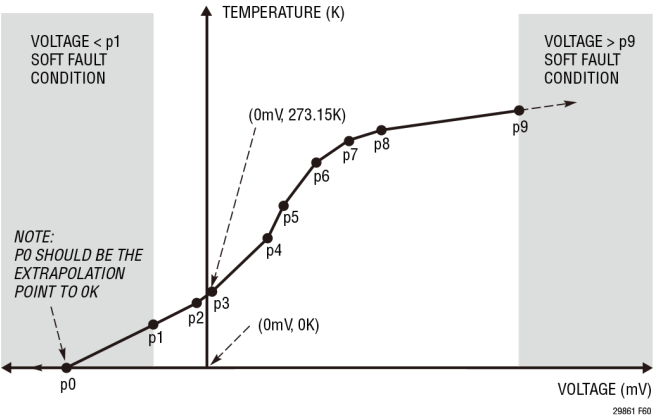
图 60. 定制热电偶示例 (mV 与开尔文的关系)
