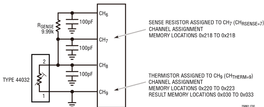
图 30. 差分热敏电阻示例
