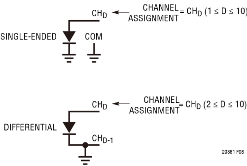
图 8. 二极管通道分配约定
