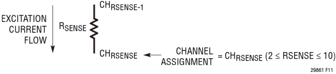
图 11. 二线式 RTD 检测电阻通道分配约定
