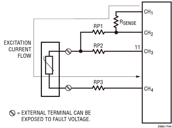
图 44. 带保护电阻的热敏电阻
