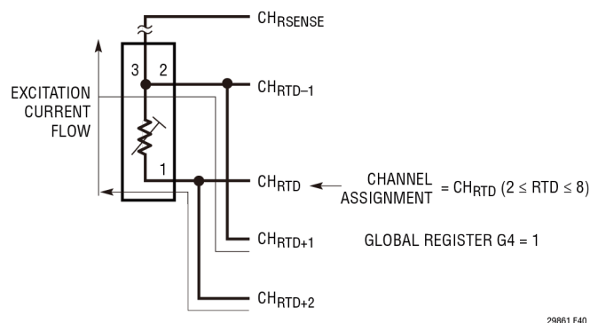
图 40. 三线式 RTD 开尔文电流模式通道分配约定 ( G4 = 1 )
