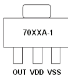
SOT89
