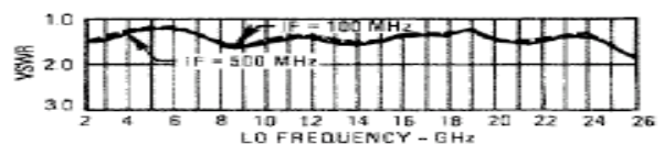
I-Port VSWR
