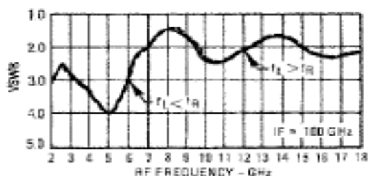
R-Port VSWR
