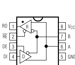
DIP/SO
