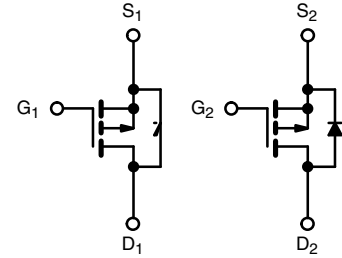
P-Channel MOSFET
