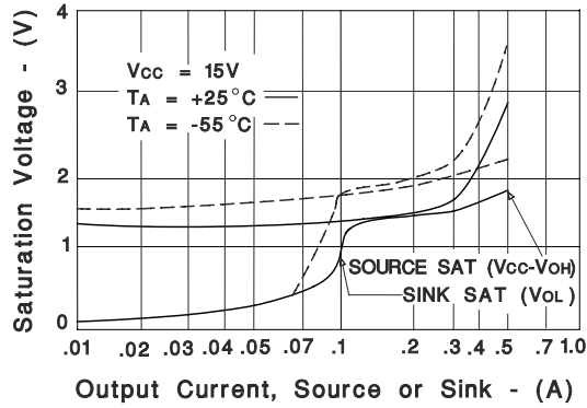
图 6-1. 输出饱和特性
