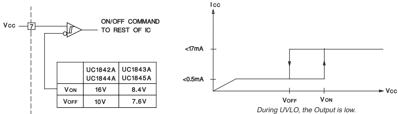
图 7-3. 欠压锁定
