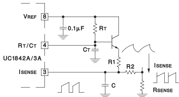
图 7-7. 斜率补偿
