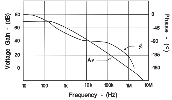
图 6-2. 误差放大器开环频率响应
