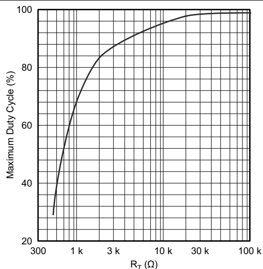
图 7-5. 最大占空比与时序电阻之间的关系
