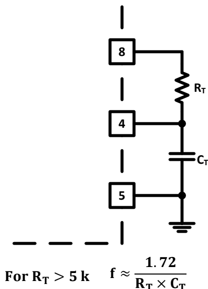
图 7-6. 振荡器选择
