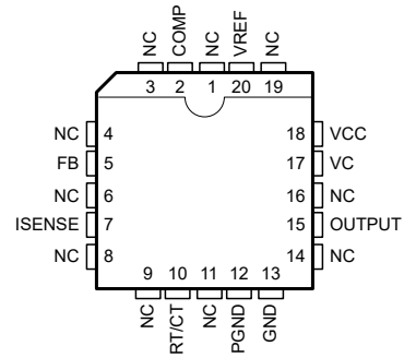
图 5-2. LCCC 和 PLCC 封装，20 引脚 FK 和 FN (顶视图)
