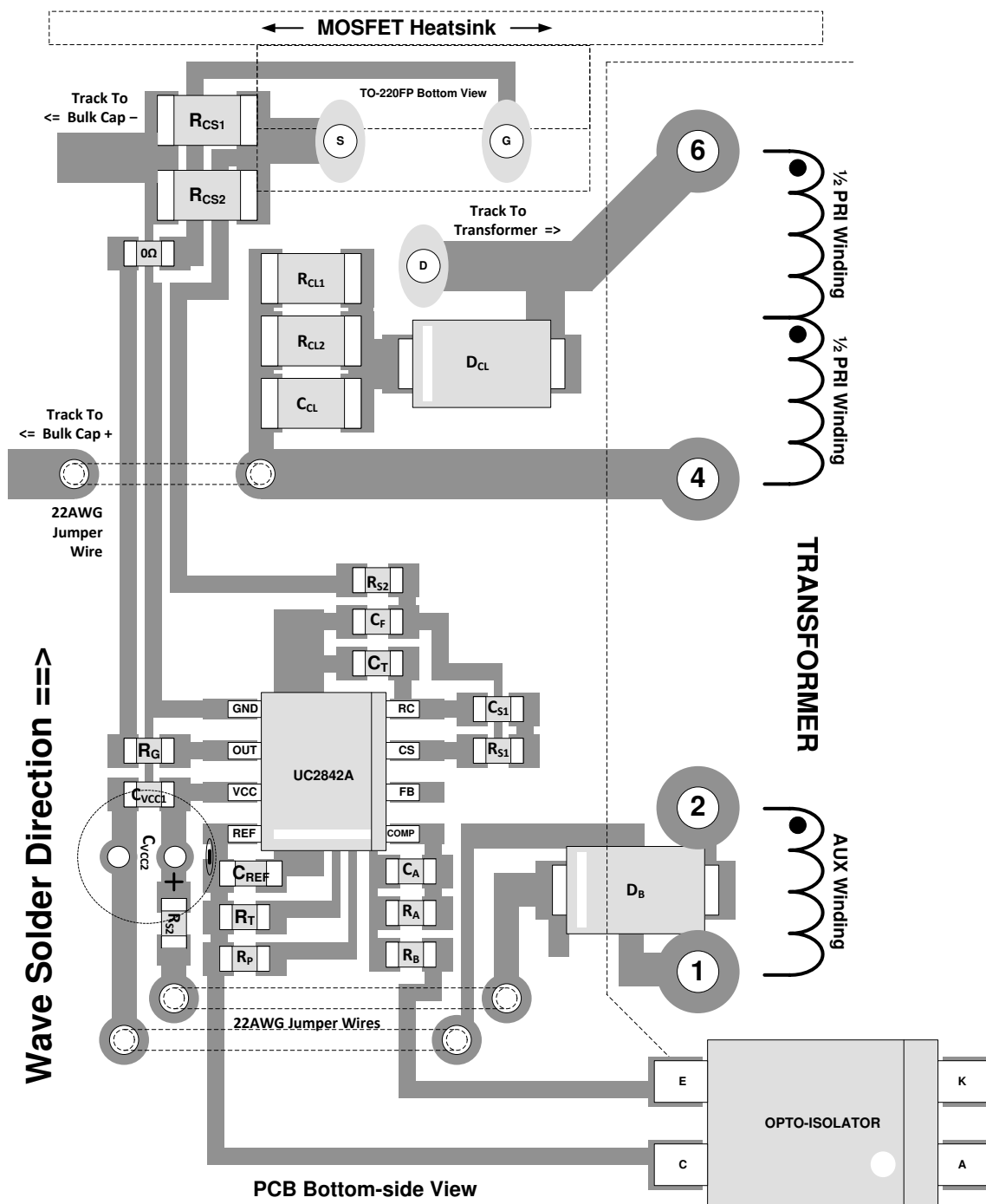
图 10-1. 布局图
