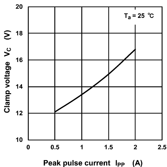
Fig. 9.1 V_C - I_{PP}
