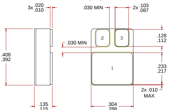
SMD.5 (S.5)
