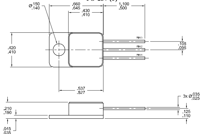
TO-257 (J)
