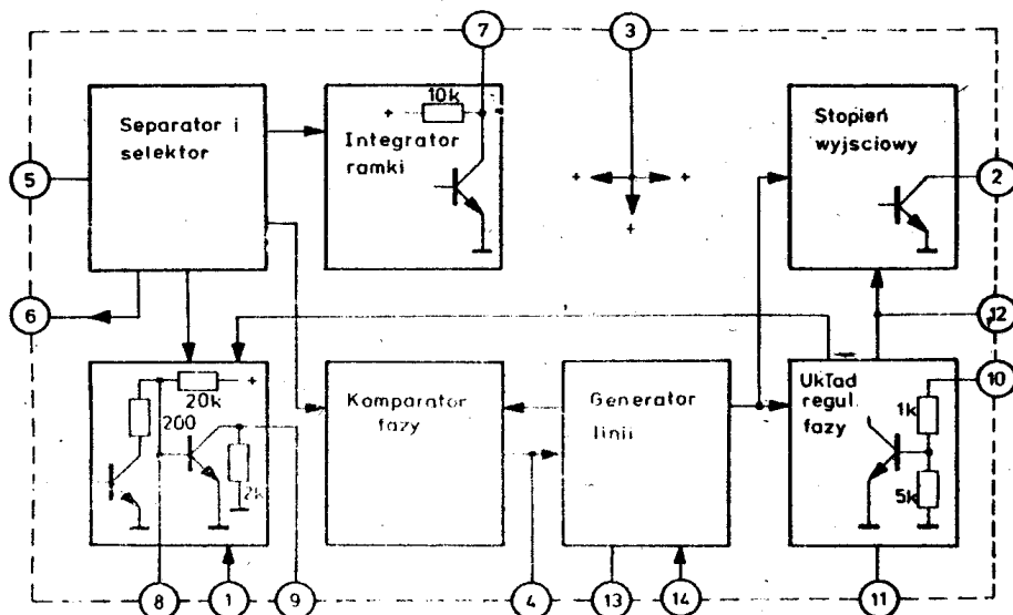
Schemat blokowy
