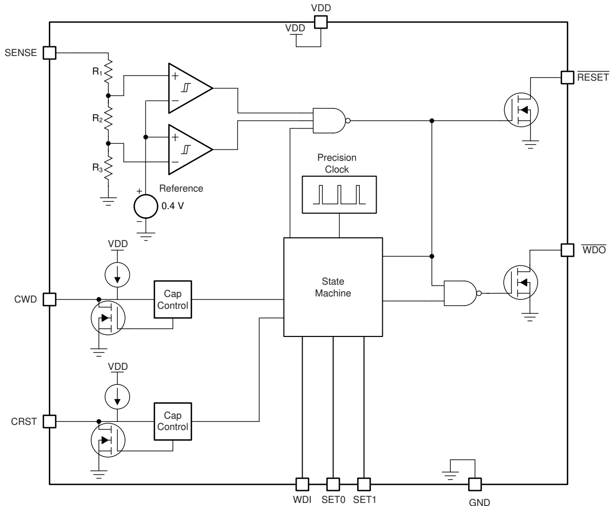
图 7-1. Fixed Version Block Diagram
