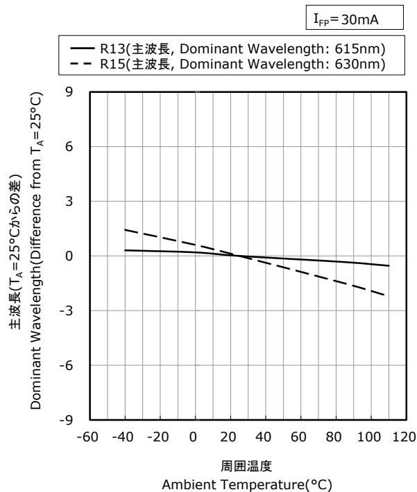
周囲温度-主波長( T_A=25^\circ\text{C} からの差)特性 Ambient Temperature vs Dominant Wavelength (Difference from T_A=25^\circ\text{C} )
